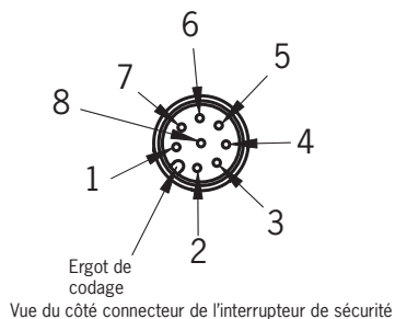
Fig. 2 : Affectation des broches interrupteur de sécurité CES-AR-C01
