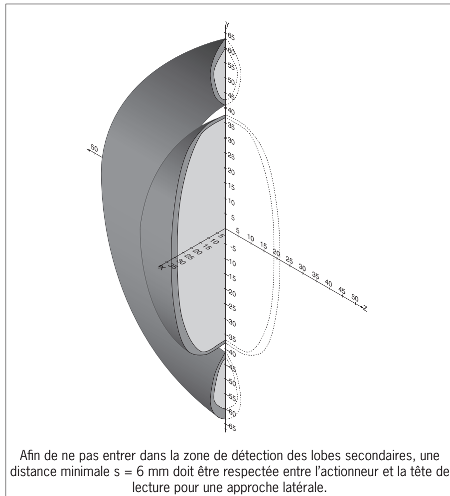
Fig. 9 : Zone de détection type
