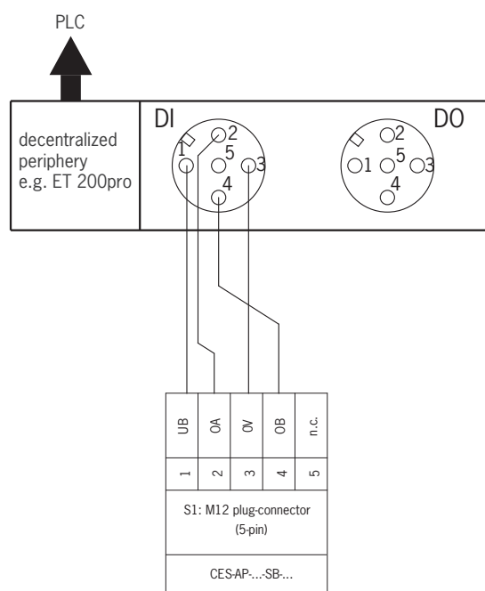
Fig. 4 : Exemple de raccordement version pour modules d'interfaces décentralisées
