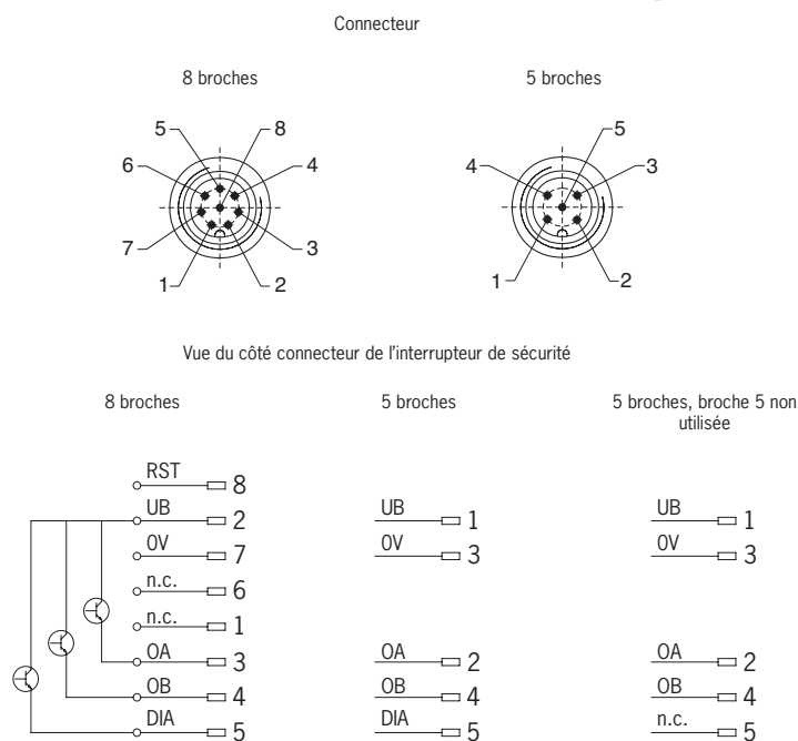
Fig. 1 : Affectation des broches interrupteur de sécurité CES-AP-C01
