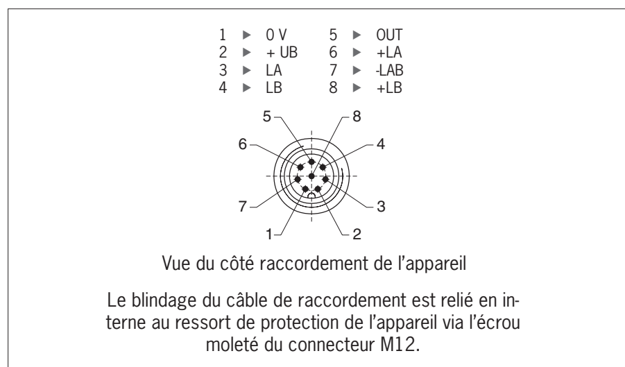
Fig. 1 : Affectation des broches interrupteur de sécurité CES-A-.5
