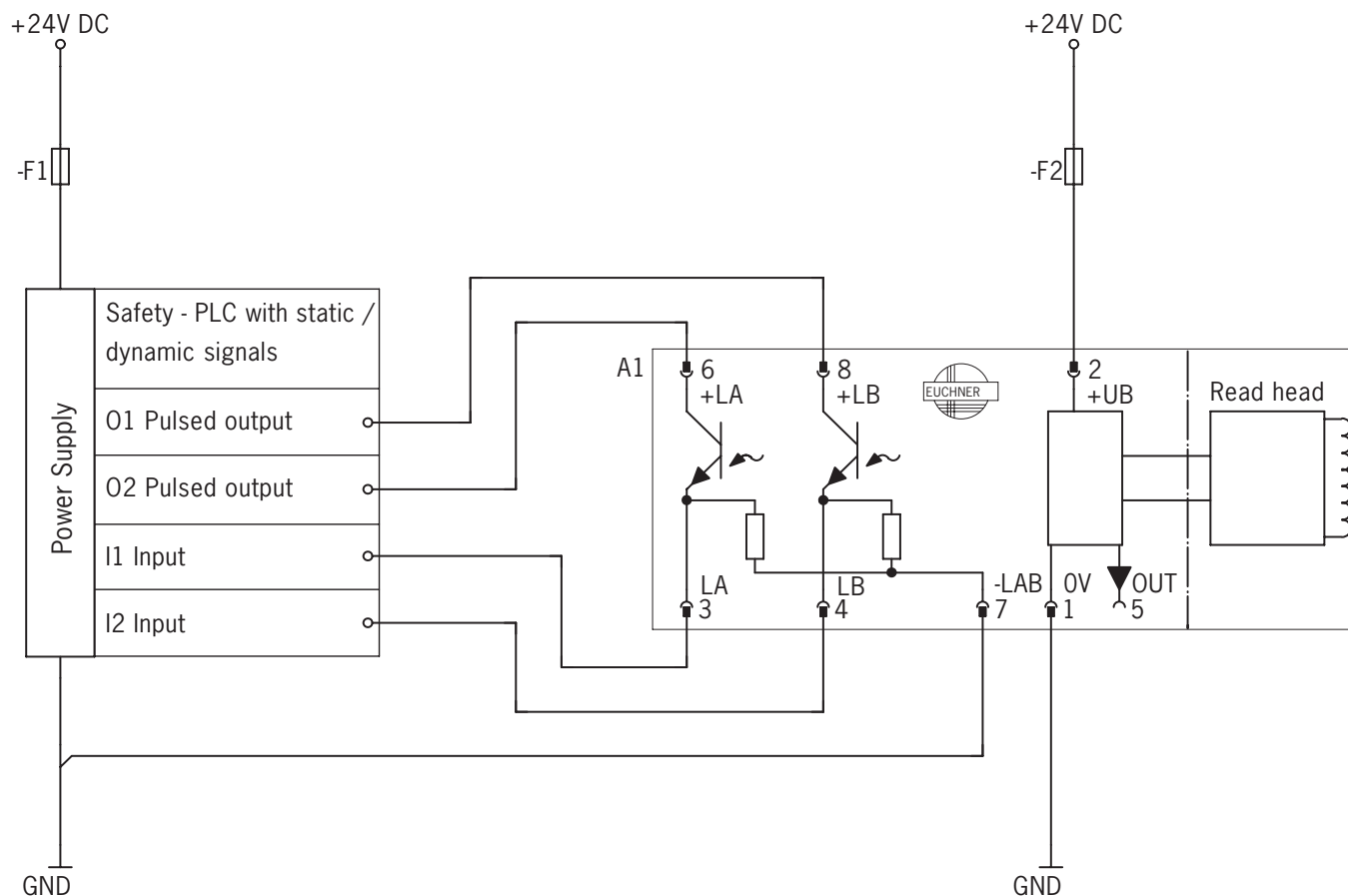
Fig. 2 : Exemple de raccordement CES-A.5
