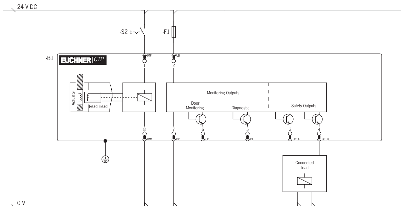
Figure 3 : Exemple de raccordement, version avec connecteur M12
