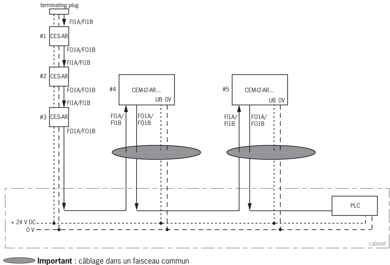
Fig. 7 : Câblage central dans un système AR au niveau de l'armoire
