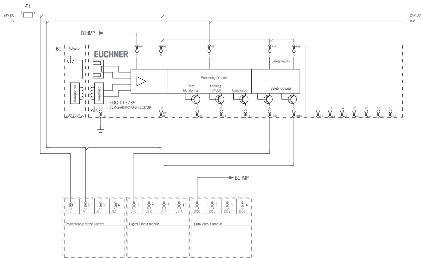
Fig. 8 : Exemple de raccordement à ET200
