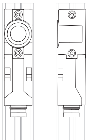
Fig. 1 : Orientations de montage avec fixation frontale ou latérale
