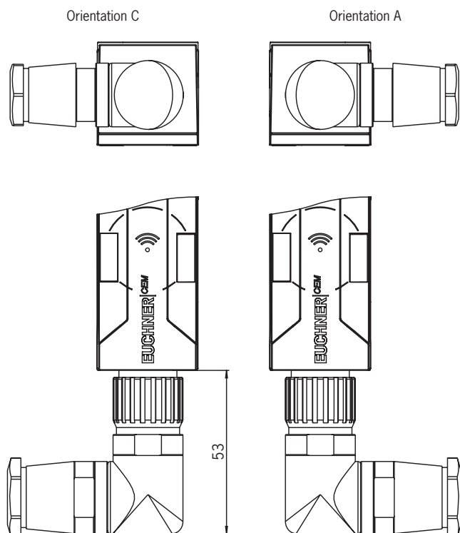
Connecteur M23
