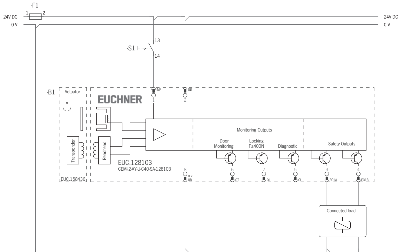
Fig. 5 : Exemple de raccordement pour CEM-AY ; version avec connecteur M12
