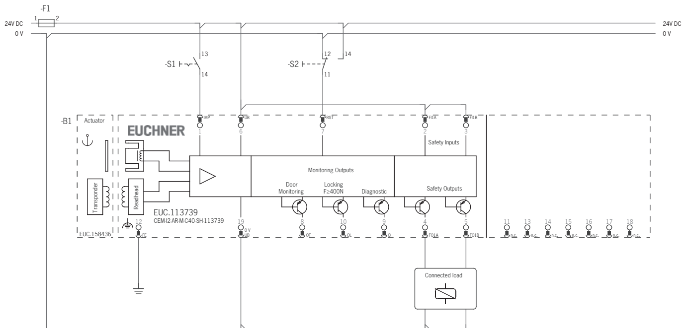
Fig. 4 : Exemple de raccordement interrupteur individuel CEM-AR ; version avec connecteur M23
