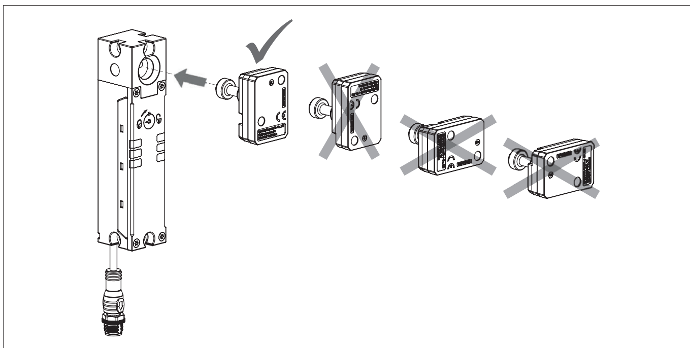
Fig. 2 : Orientation actionneur
