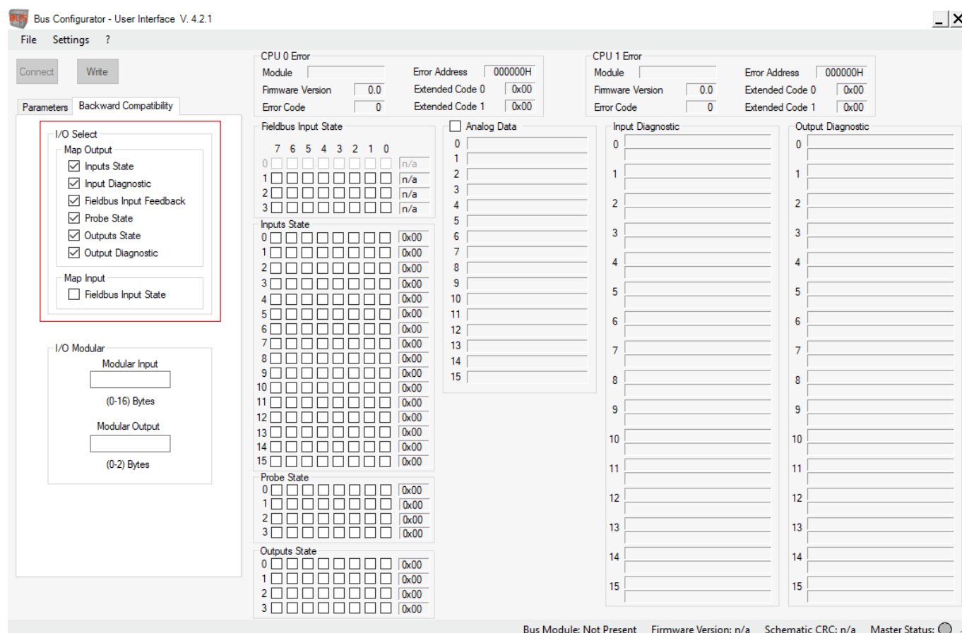
Fig. 7 : Bus Configurator – User Interface, mode de compatibilité
