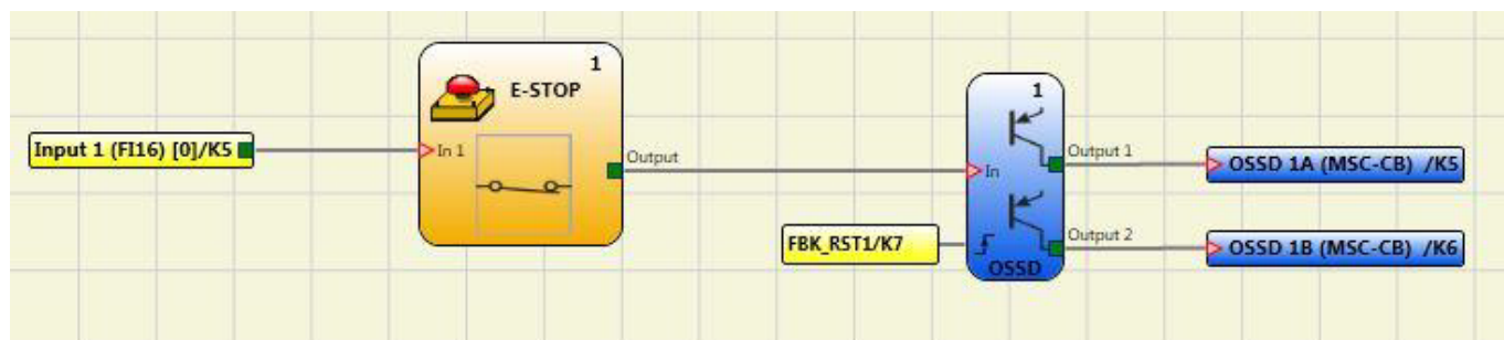
Fig. 11 : Diagnostic-exemple 3 avec fonction de réinitialisation manuelle
