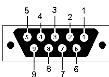
Connecteur femelle DB9 (vue avant)
