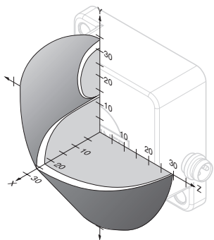
avec actionneur CES-A-BQA sur analyseur CES-A-UBA-01B
