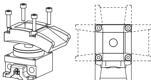
Fig. 1: Modifica della direzione di azionamento
