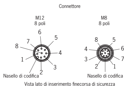
Fig. 2: Collegamenti finecorsa di sicurezza CES-I-AR
