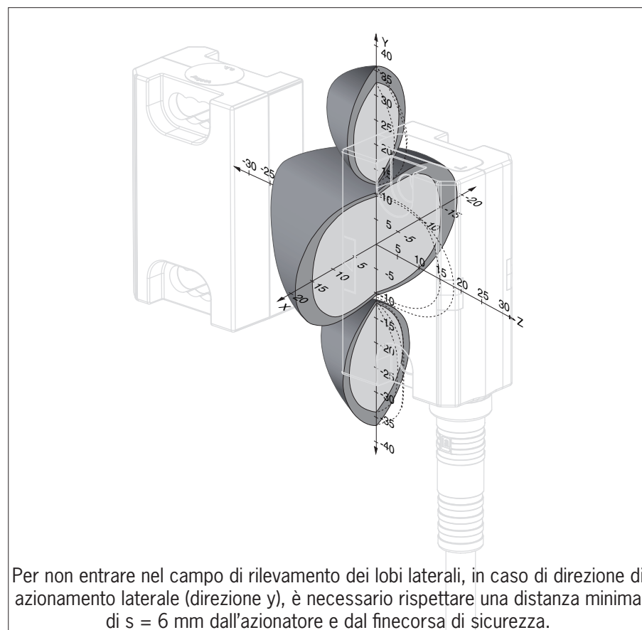
Fig. 6: Campo di rilevamento tipico
