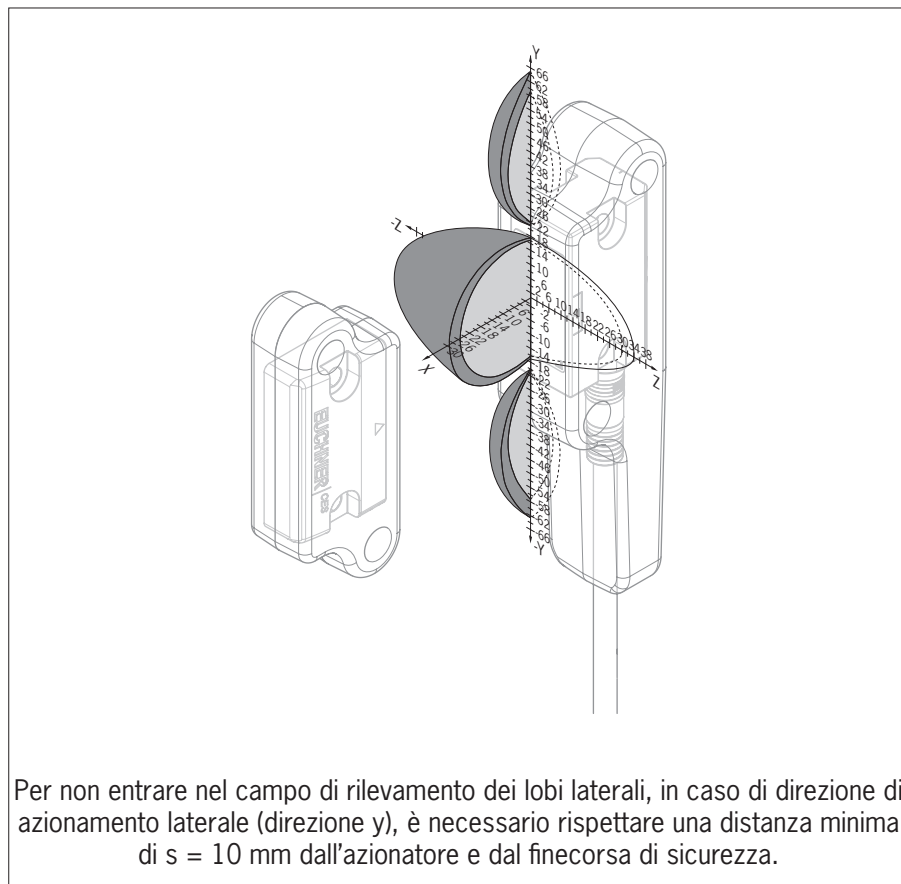
Fig. 7: Campo di rilevamento tipico
