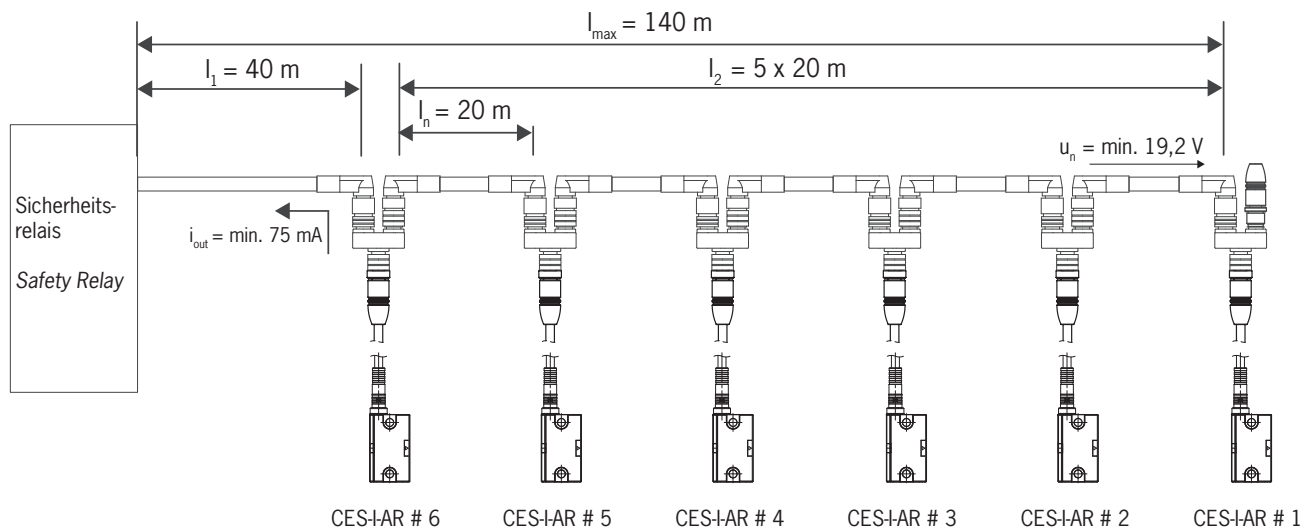
Fig. 1: Esempio di collegamento con sei CES-I-AR
