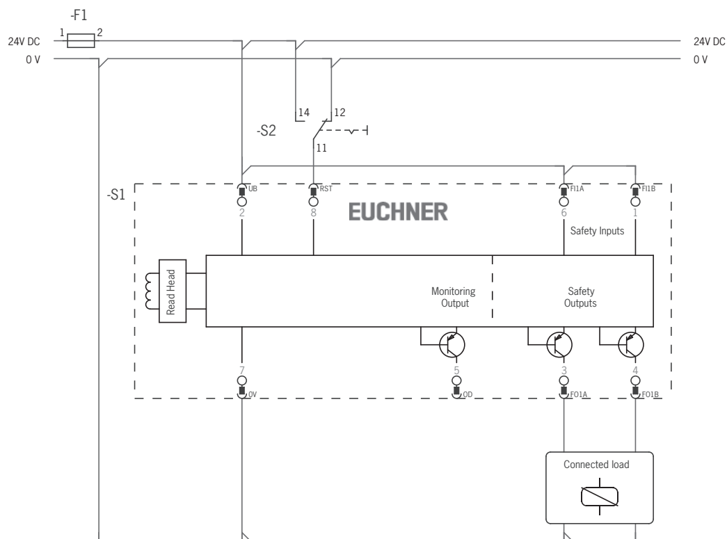
Fig. 3: Esempio di collegamento per funzionamento singolo di un CES-I-AR-...
