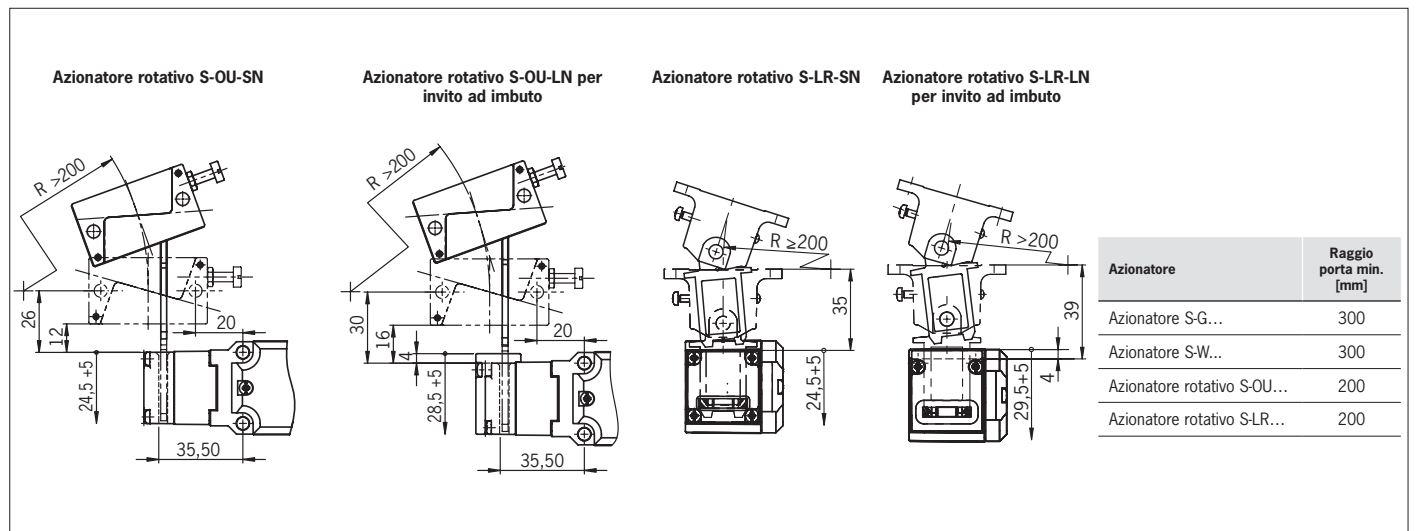
Fig. 4: Raggi porta minimi
