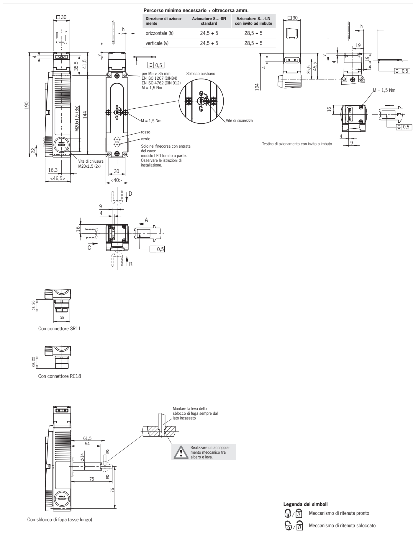
Fig. 2: Dimensioni STA... senza invito ad imbuto e STA... con invito ad imbuto
