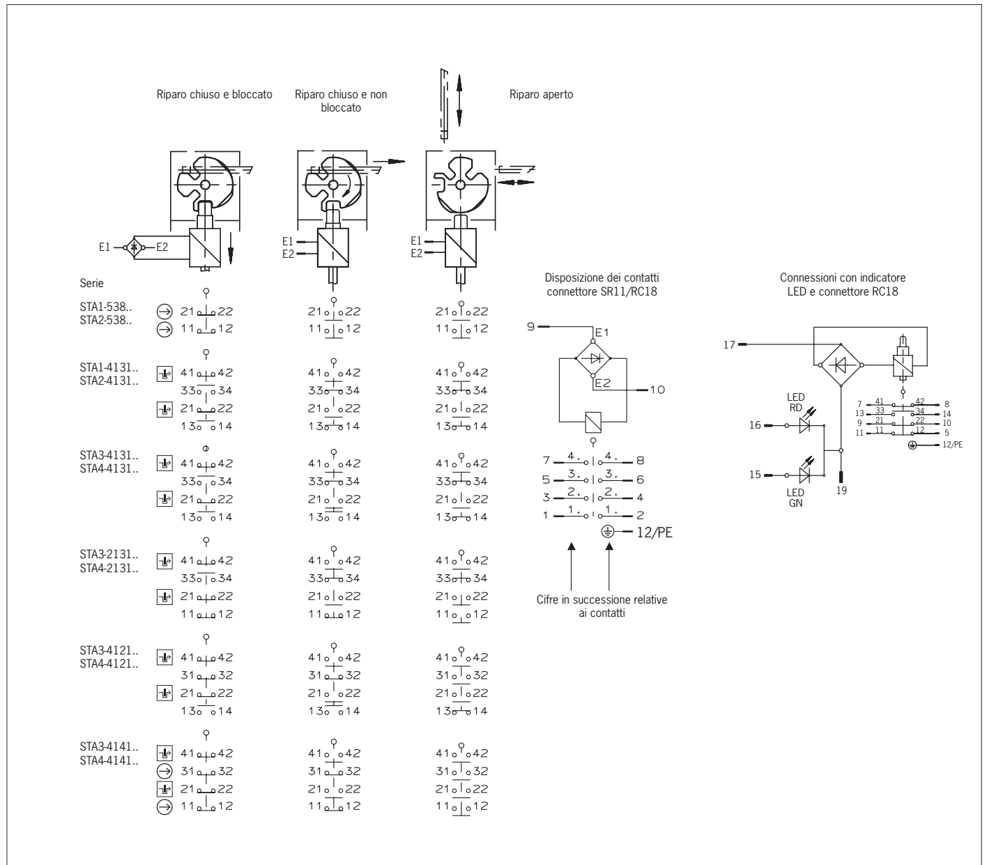
Fig. 3: Microinterruttori e commutazioni
