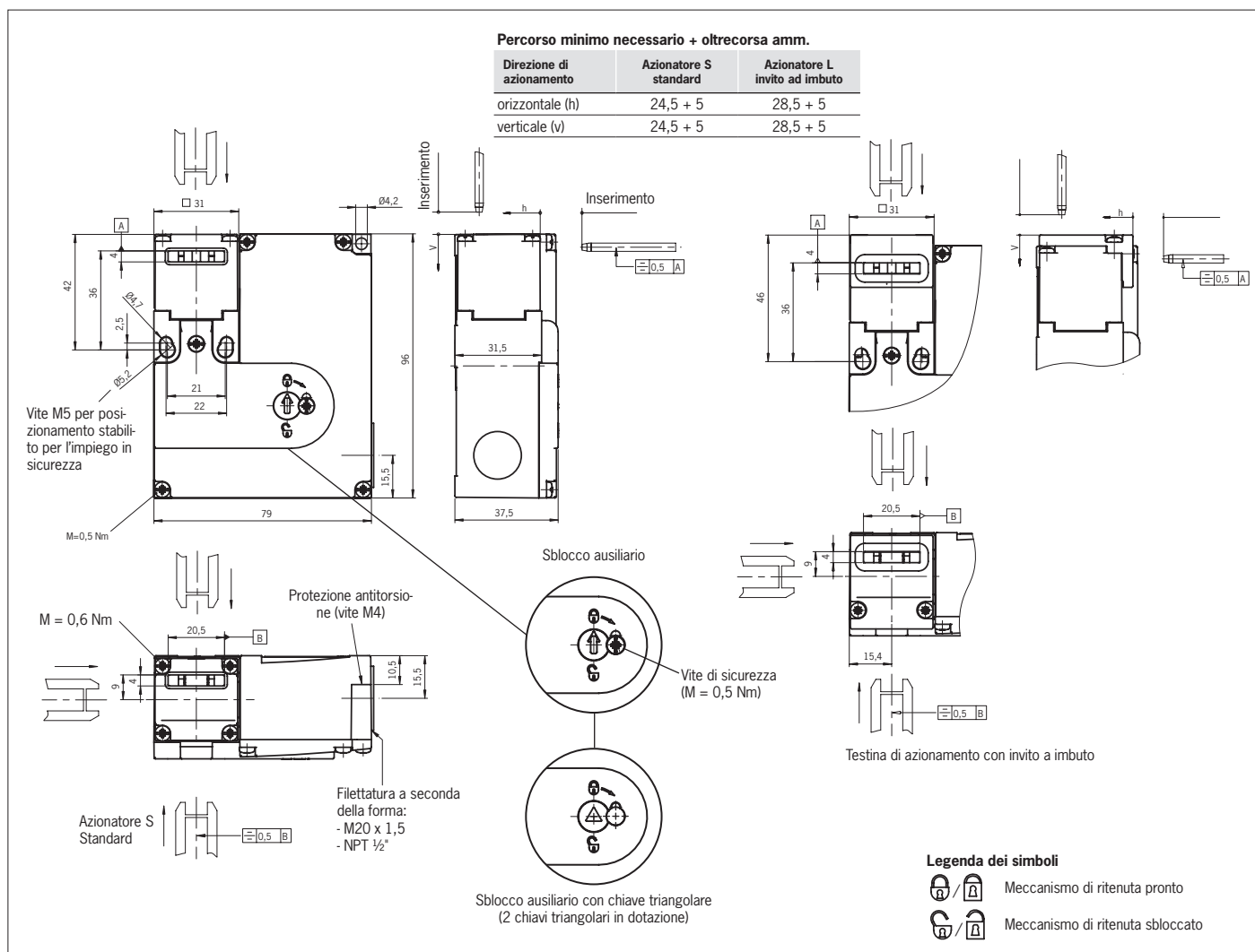
Fig. 6: Dimensioni STM... senza invito ad imbuto e STM... con invito ad imbuto
