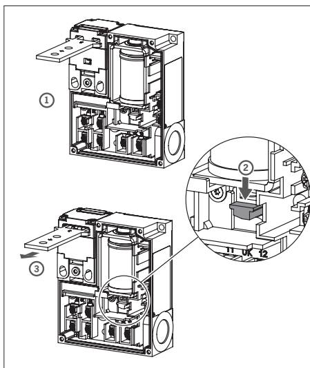
Fig. 3: Rimuovere l'azionatore
