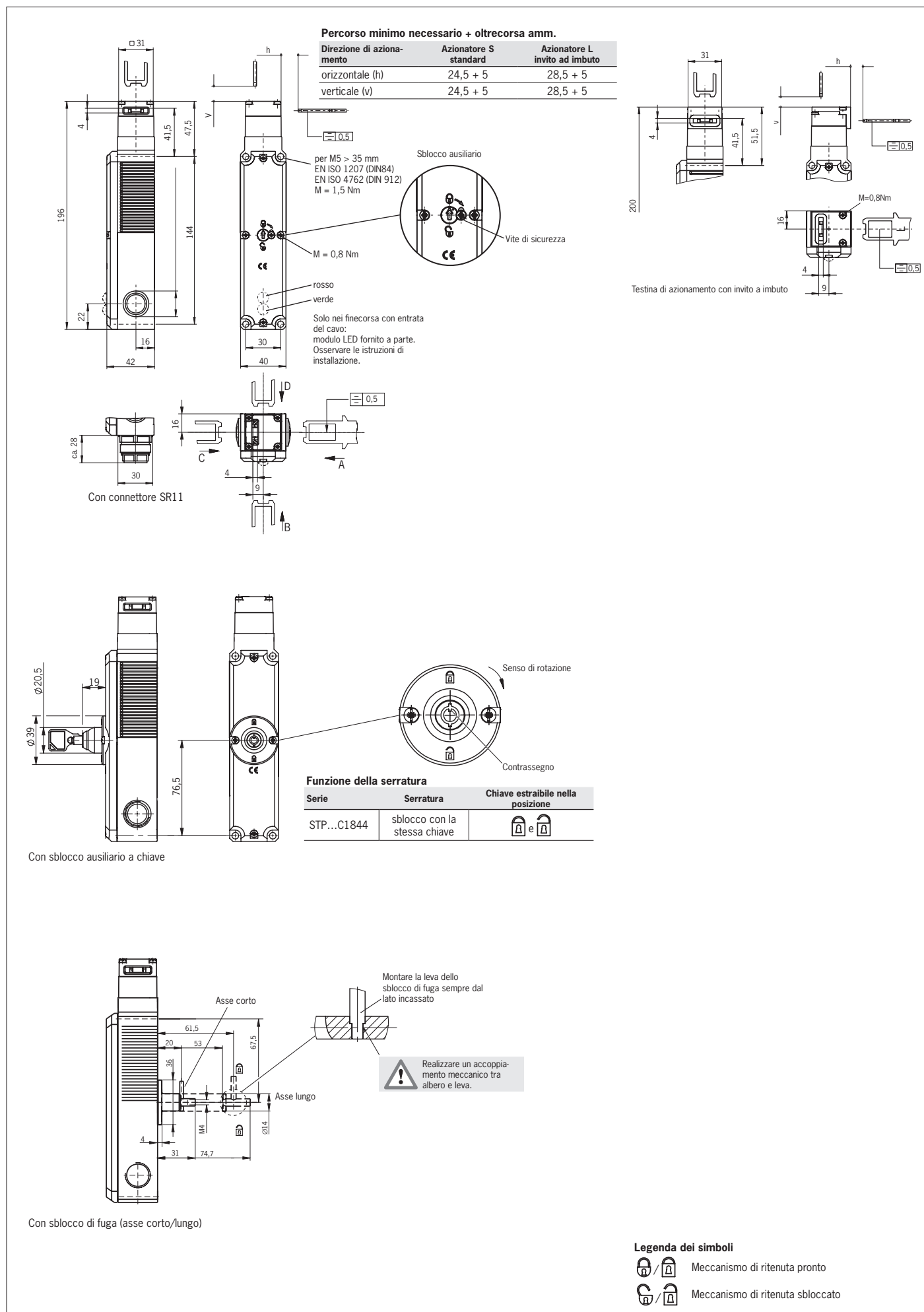
Fig. 2: Dimensioni STP... senza invito ad imbuto e STP... con invito ad imbuto
