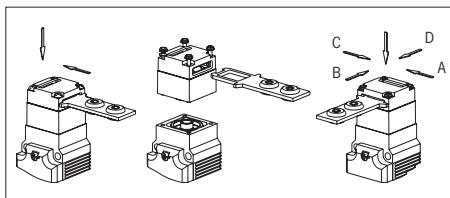
Fig. 1: Modifica della direzione di azionamento
