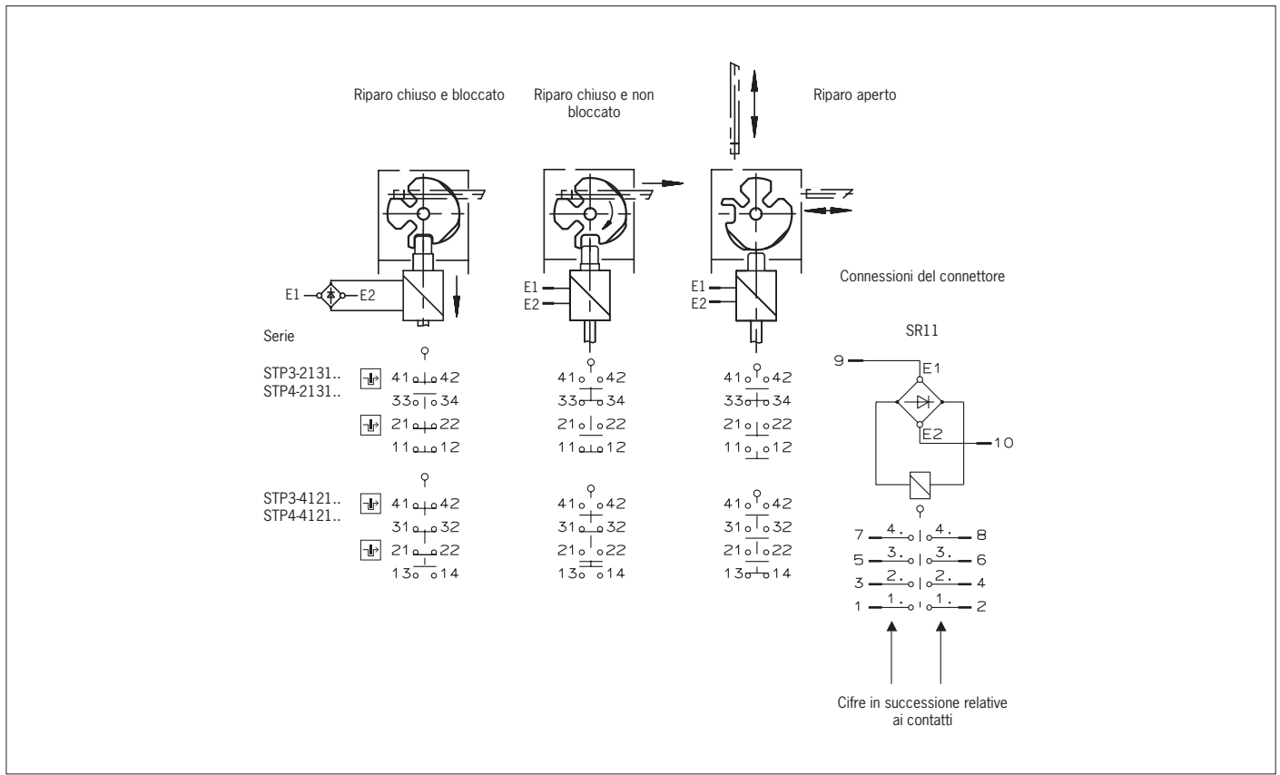
Fig. 3: Microinterruttori e commutazioni
