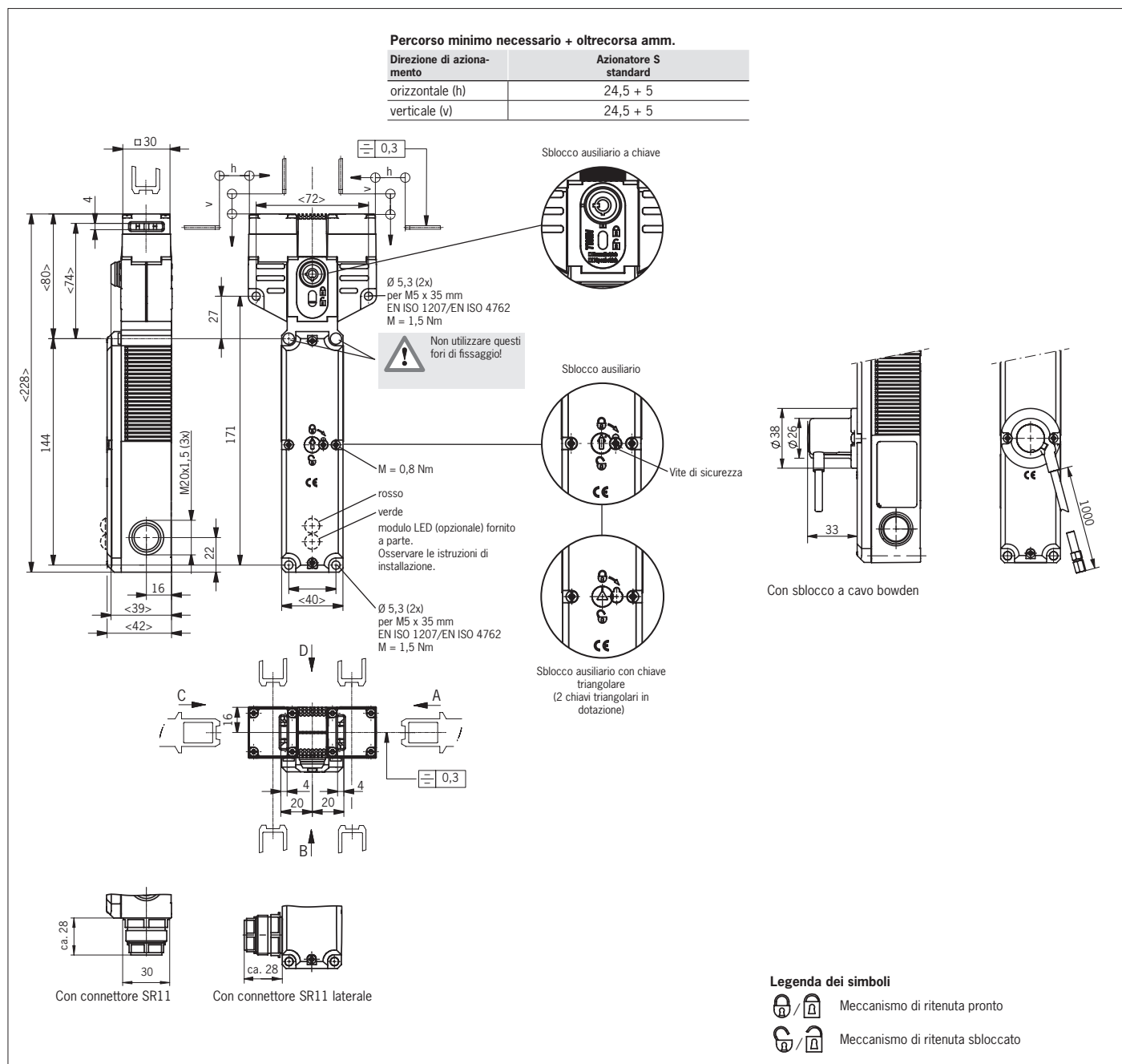
Fig. 3: Dimensioni STP-TW...
