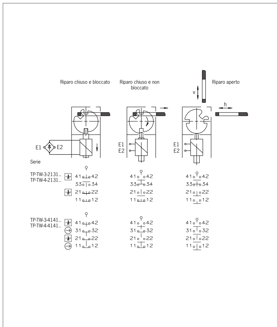
Fig. 4: Microinterruttori e commutazioni
