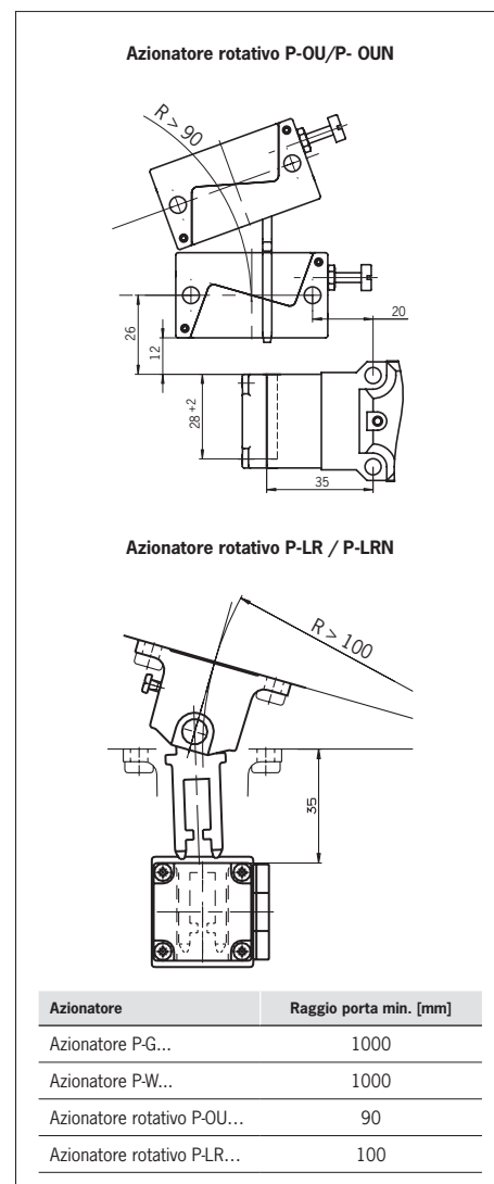
Fig. 5: Raggi porta minimi
