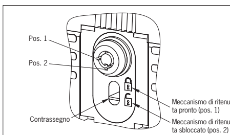
Fig. 1: Sblocco ausiliario a chiave e indicatore
