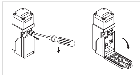
Fig. 3: Apertura del finecorsa di sicurezza
