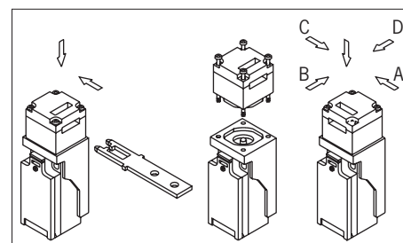
Fig. 1: Modifica della direzione di azionamento
