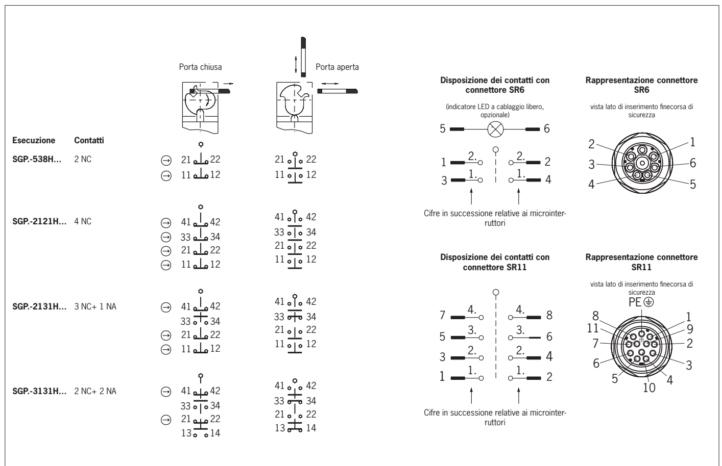
Fig. 2: Microinterruttori e commutazioni
