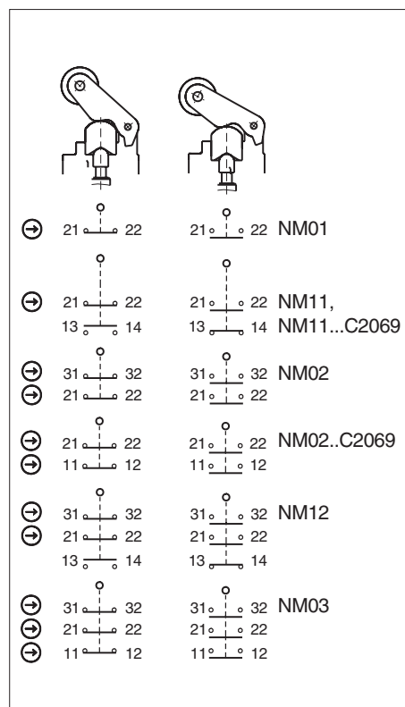
Fig. 3: Microinterruttori e commutazioni
