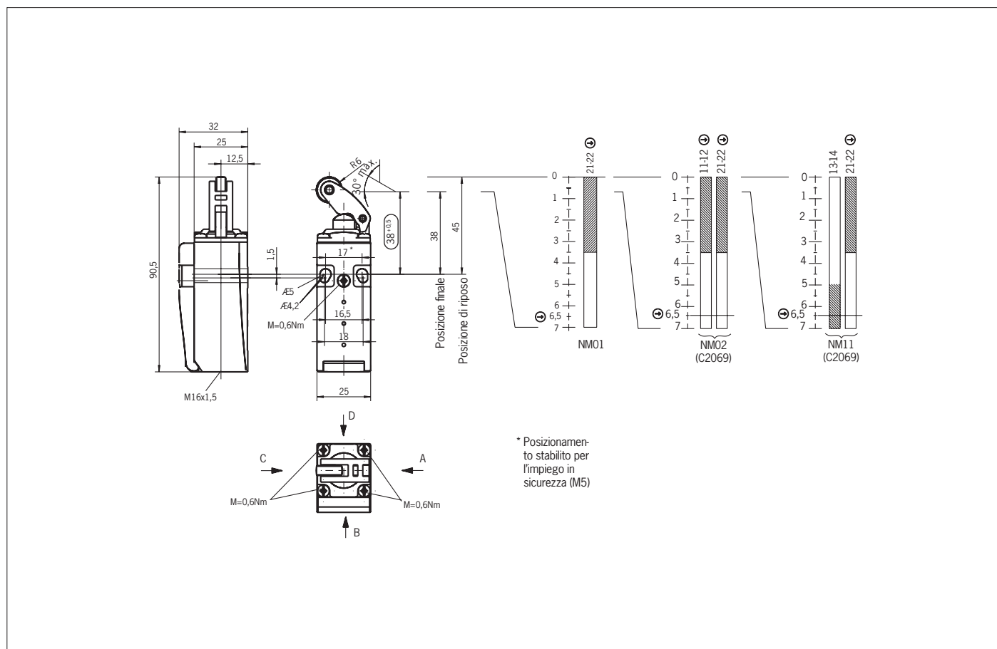
Fig. 5: Dimensioni e diagrammi di funzionamento NM01KB, NM...C2069
