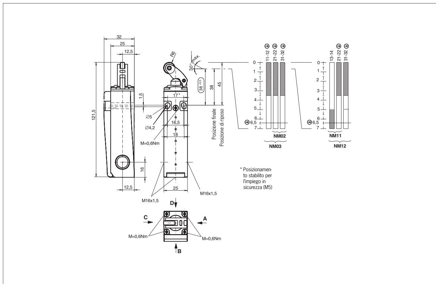
Fig. 4: Dimensioni e diagrammi di funzionamento NM11KB / NM02KB / NM12KB / NM03KB
