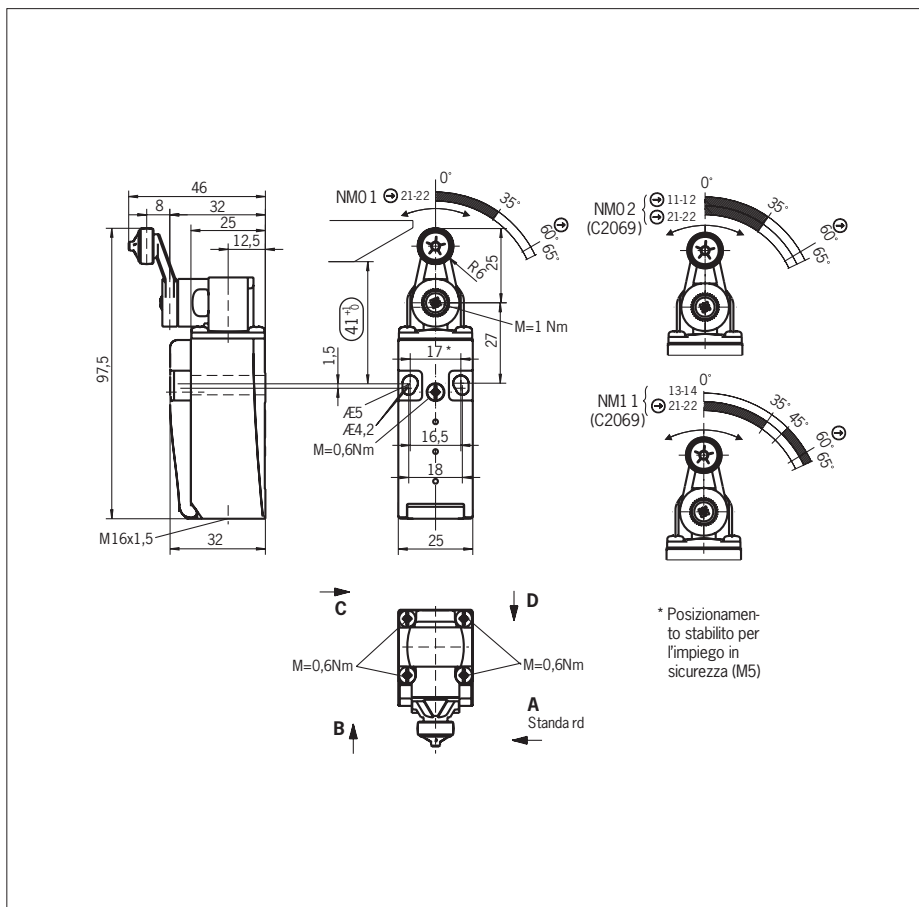
Fig. 6: Dimensioni e diagrammi di funzionamento NM01HB, NM...C2069
