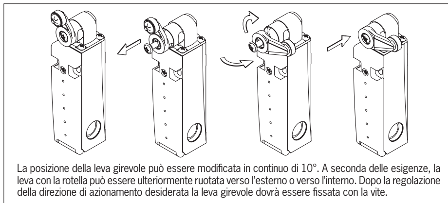
Fig. 3: Modifica della posizione della leva girevole
