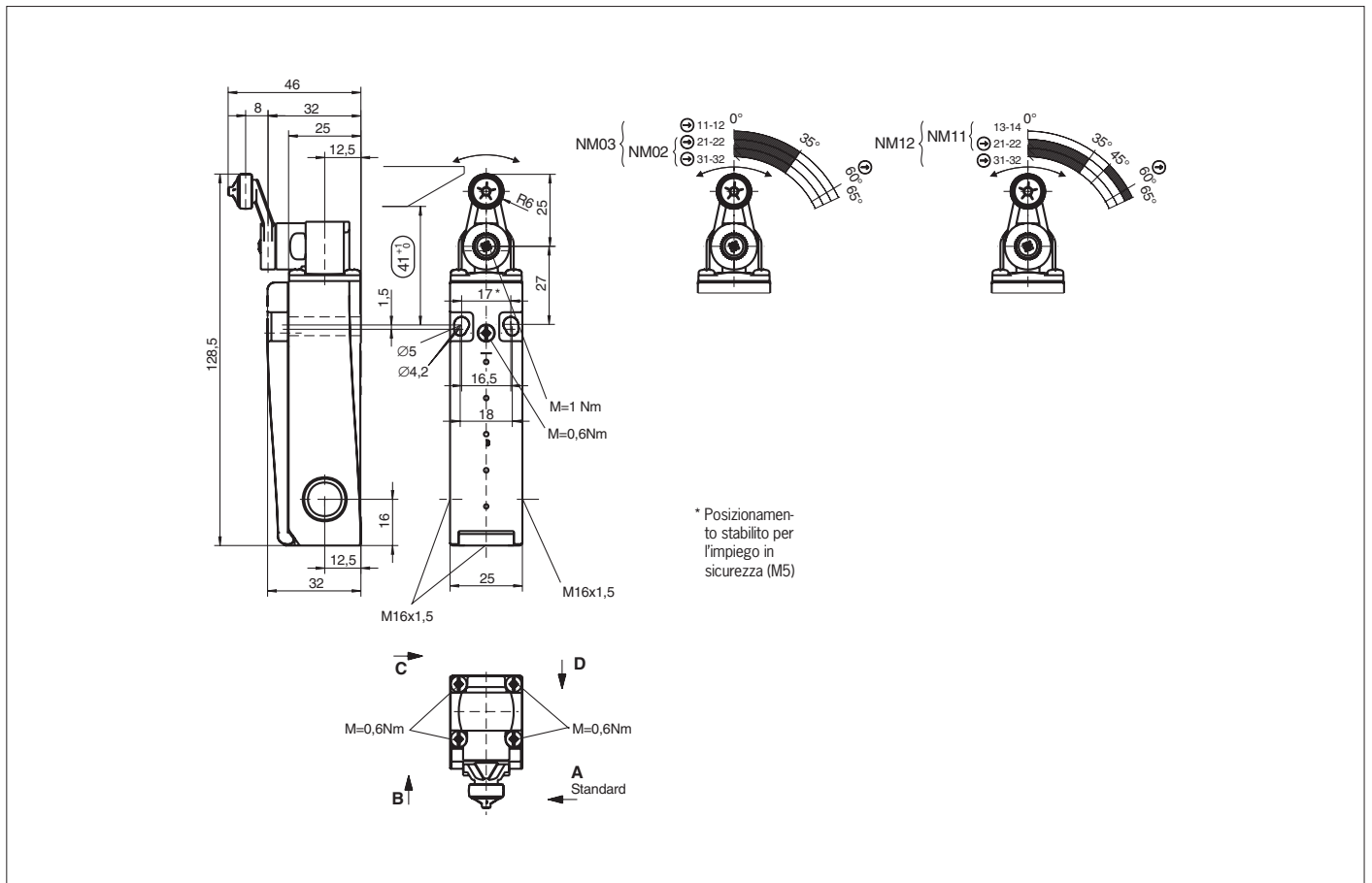
Fig. 5: Dimensioni e diagrammi di funzionamento NM11HB / NM02HB / NM12HB / NM03HB
