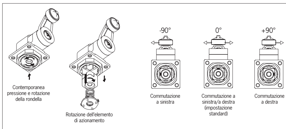
Fig. 4: Modifica della direzione di commutazione
