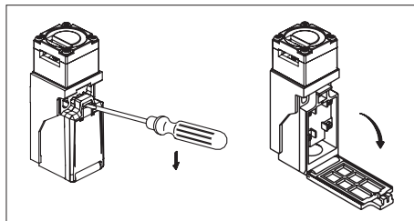
Fig. 3: Apertura del finecorsa di sicurezza
