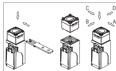
Fig. 1: Modifica della direzione di azionamento
