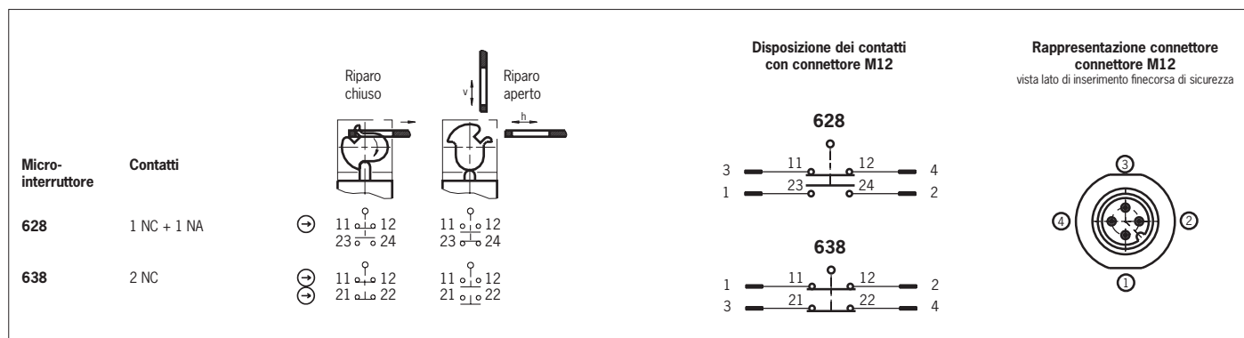
Fig. 4: Microinterruttori e commutazioni
