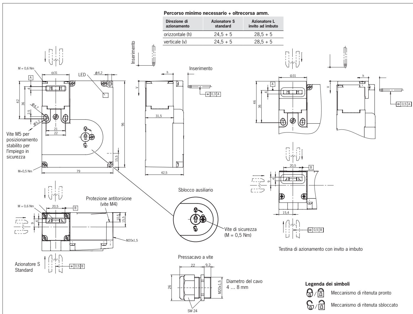
Fig. 6: Dimensioni STM Pro senza invito ad imbuto e STM Pro con invito ad imbuto
