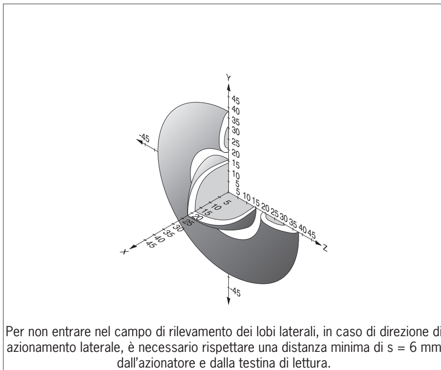
Fig. 8: Campo di rilevamento tipico
