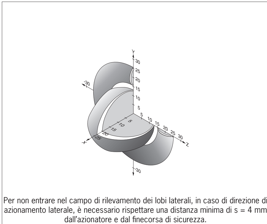
Fig. 6: Campo di rilevamento tipico
