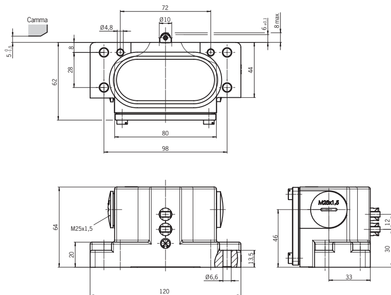
Fig. 2: Dimensioni GS...502-MC1806
