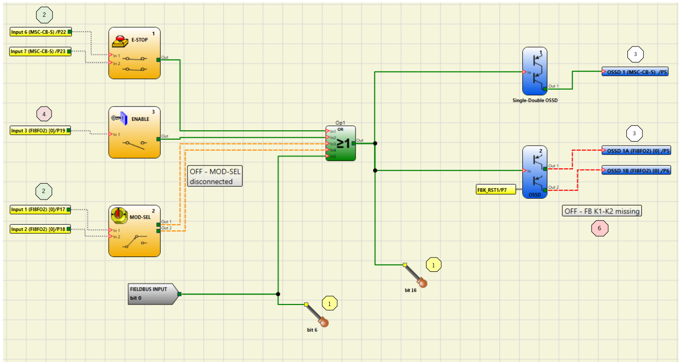
Fig. 16: Esempio di progetto su EUCHNER Safety Designer
