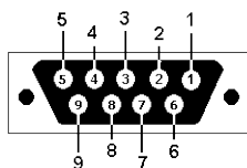
DB9 femmina (vista frontale)
