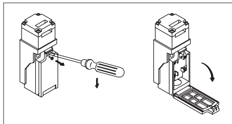
Fig. 3: Apertura del fincorsa di sicurezza
