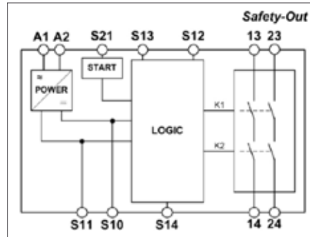
그림 1: ESM-BA2..의 블록 선도
