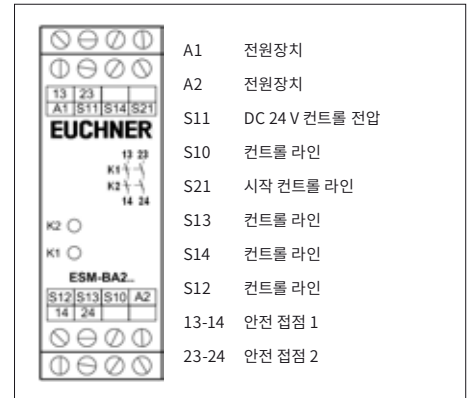
그림 3: 연결부
