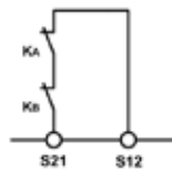
그림 13: 자동 시작 기능이 포함된 피드백 루프. 외부 연결 접점 또는 확장 모듈 모니터링
