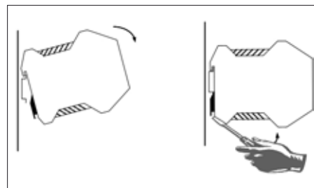
그림 2: 설치/제거
