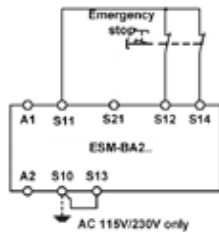
그림 6: 듀얼 채널 비상 정지 회로, 접지 오류 모니터링 포함(카테고리 3, PL d까지).
