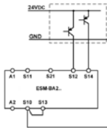
그림 9: Pnp 반도체 출력부/단락 회로 감지 장치가 있는 OSSD 출력부가 장착된 듀얼 채널 비상정지 회로(범주 4, 최대 PL e).
