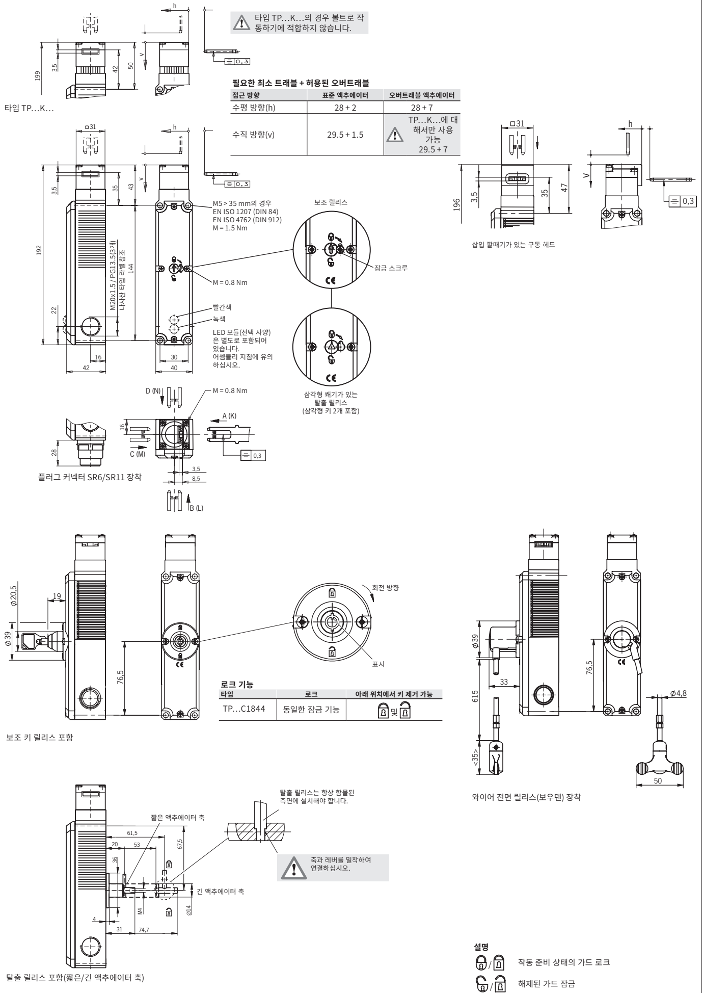
그림 2: TP...용 치수 도면
