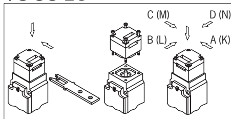
그림 1: 구동 방향 변경
