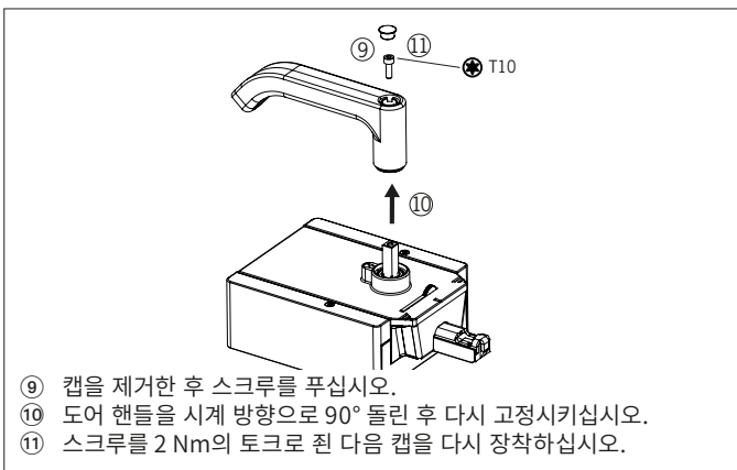
그림 15: 구동 방향 변경, 단계 ⑨ 및 ⑪
