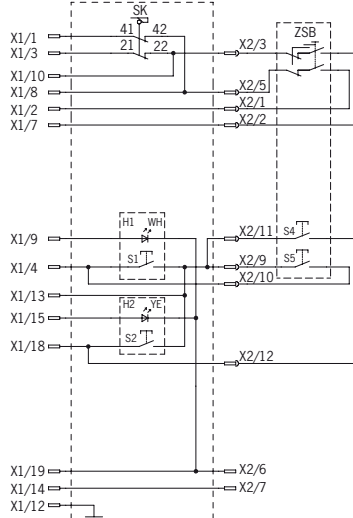
Rysunek 9: TZ..VA-C2199 z podświetlanymi przyciskami i przylączem przełącznika zgody
