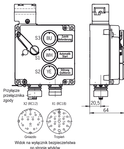
Rysunek 8: TZ..VAB-C2189/2198 ze kontrolkami/przyciskami podświetlanymi i przylączem przełącznika zgody
