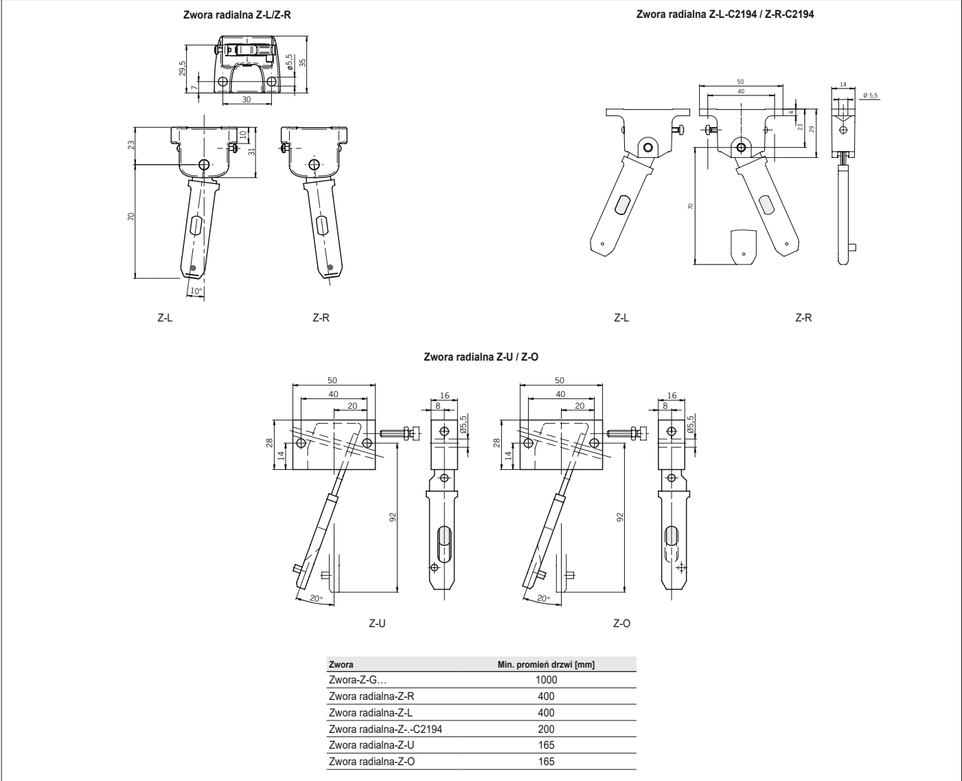
Rysunek 10: Minimalne promienie drzwi
