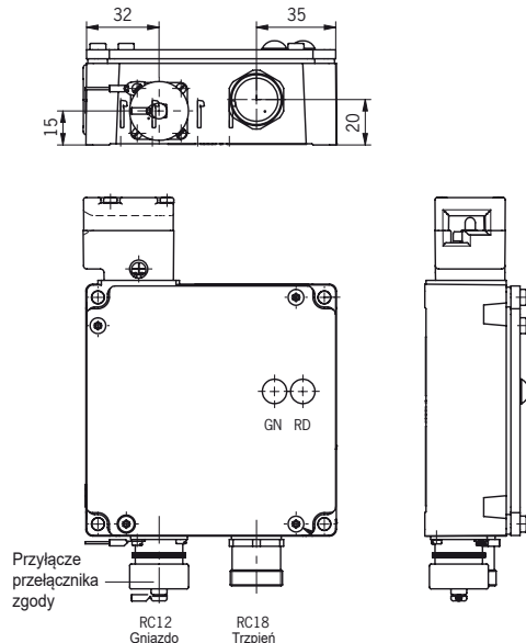
Rysunek 7: TZ..VAB-C1803 z przylączem przełącznika zgody
