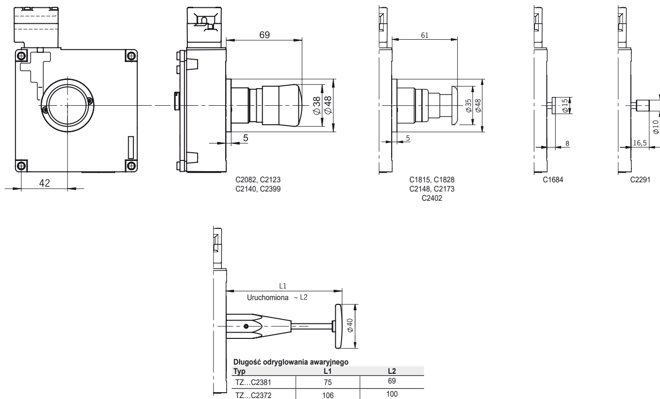
Rysunek 4: Rysunki wymiarowe odryglowań ewakuacyjnych
