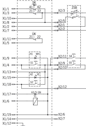
Rysunek 8: TZ..VAB-C2189/2198 ze kontrolkami/przyciskami podświetlanymi i przylączem przełącznika zgody
