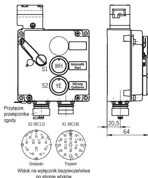
Rysunek 9: TZ..VA-C2199 z podświetlanymi przyciskami i przylączem przełącznika zgody
