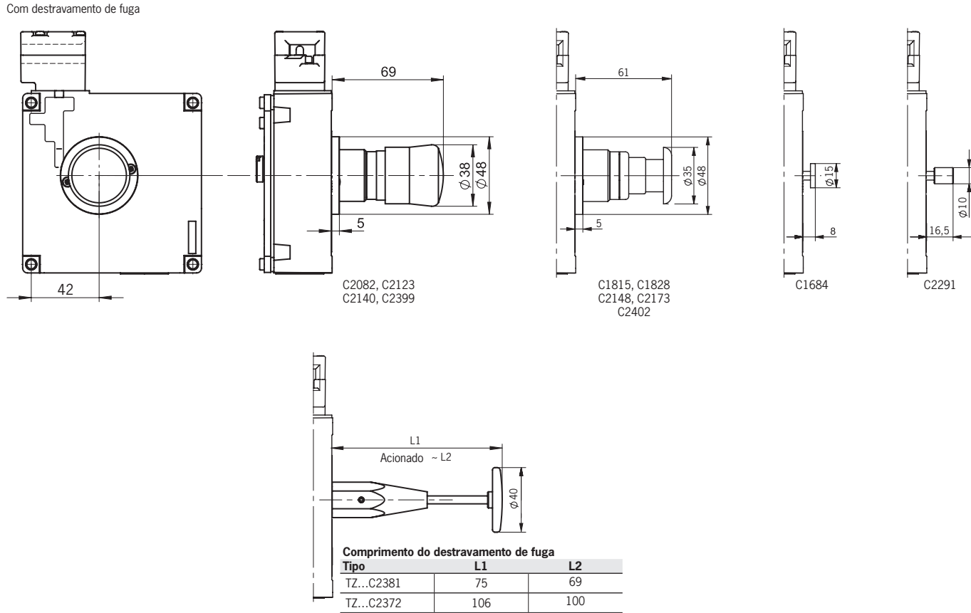
Fig. 4: Desenhos dimensionais destravamento de fuga
