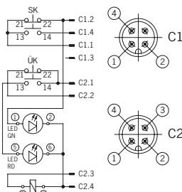
TZ.SEM4-C1888 (com conector 2 x M12, conforme DESINA)
