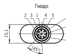
Y-образный распределитель 097627
