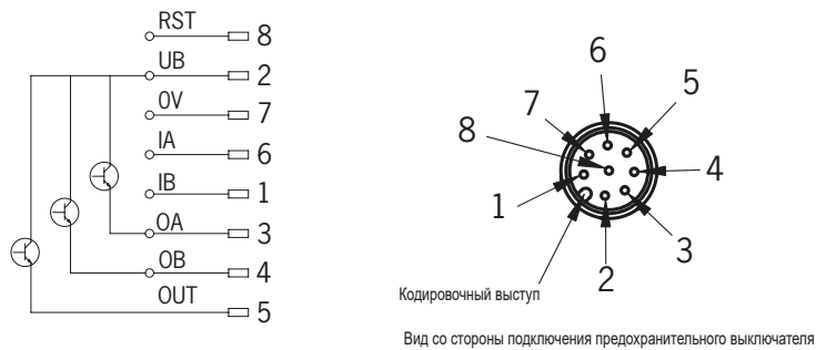
Рис. 2. Схема контактов штекерного разъема предохранительного выключателя CES-AR
