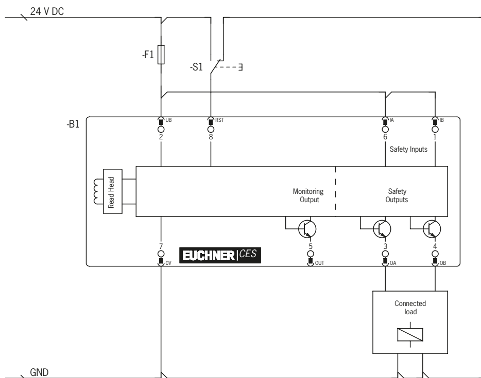
Рис. 3. Пример подключения для отдельного устройства CES-AR-...
