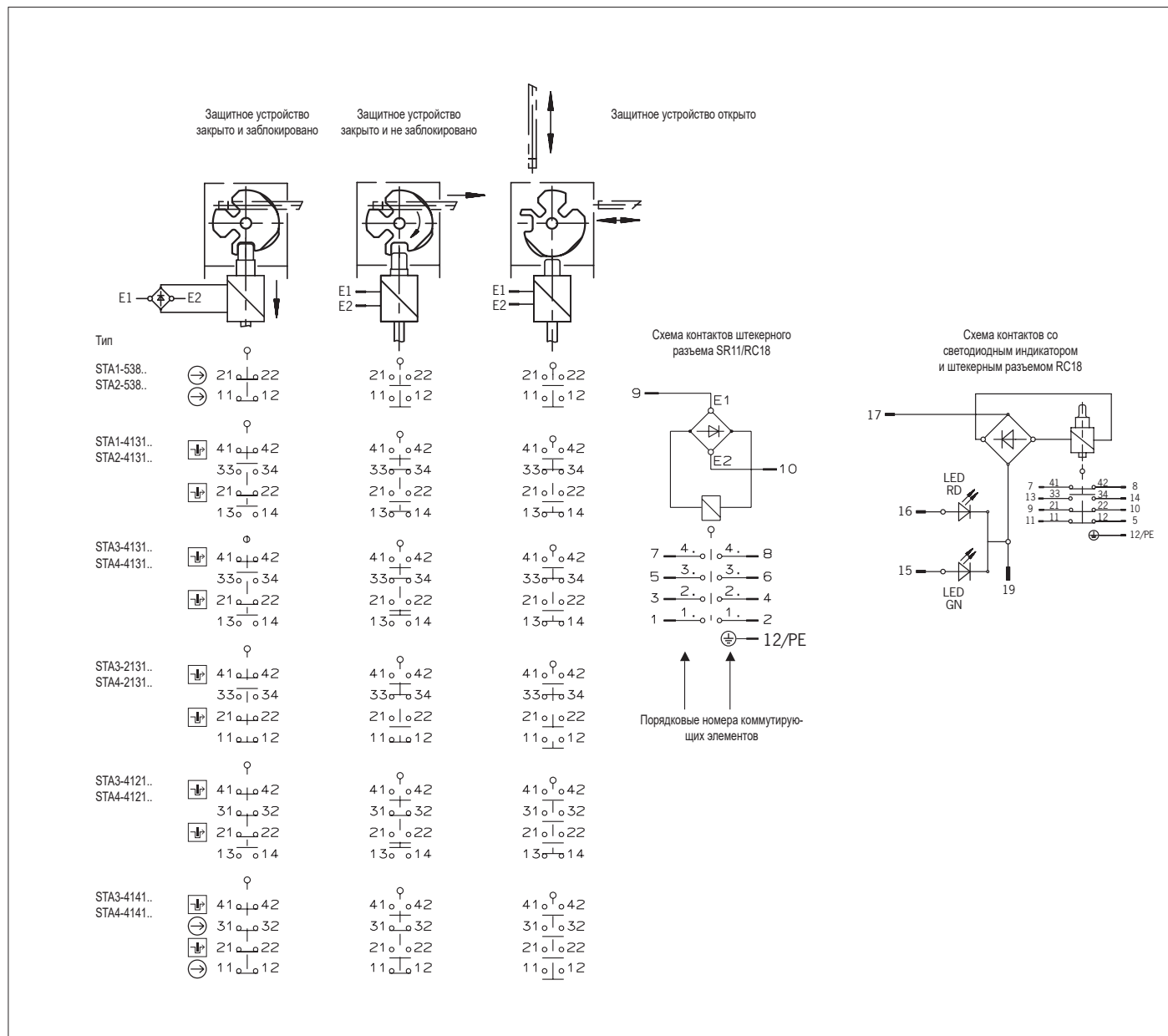
Рис. 3. Коммутирующие элементы и функции переключения
