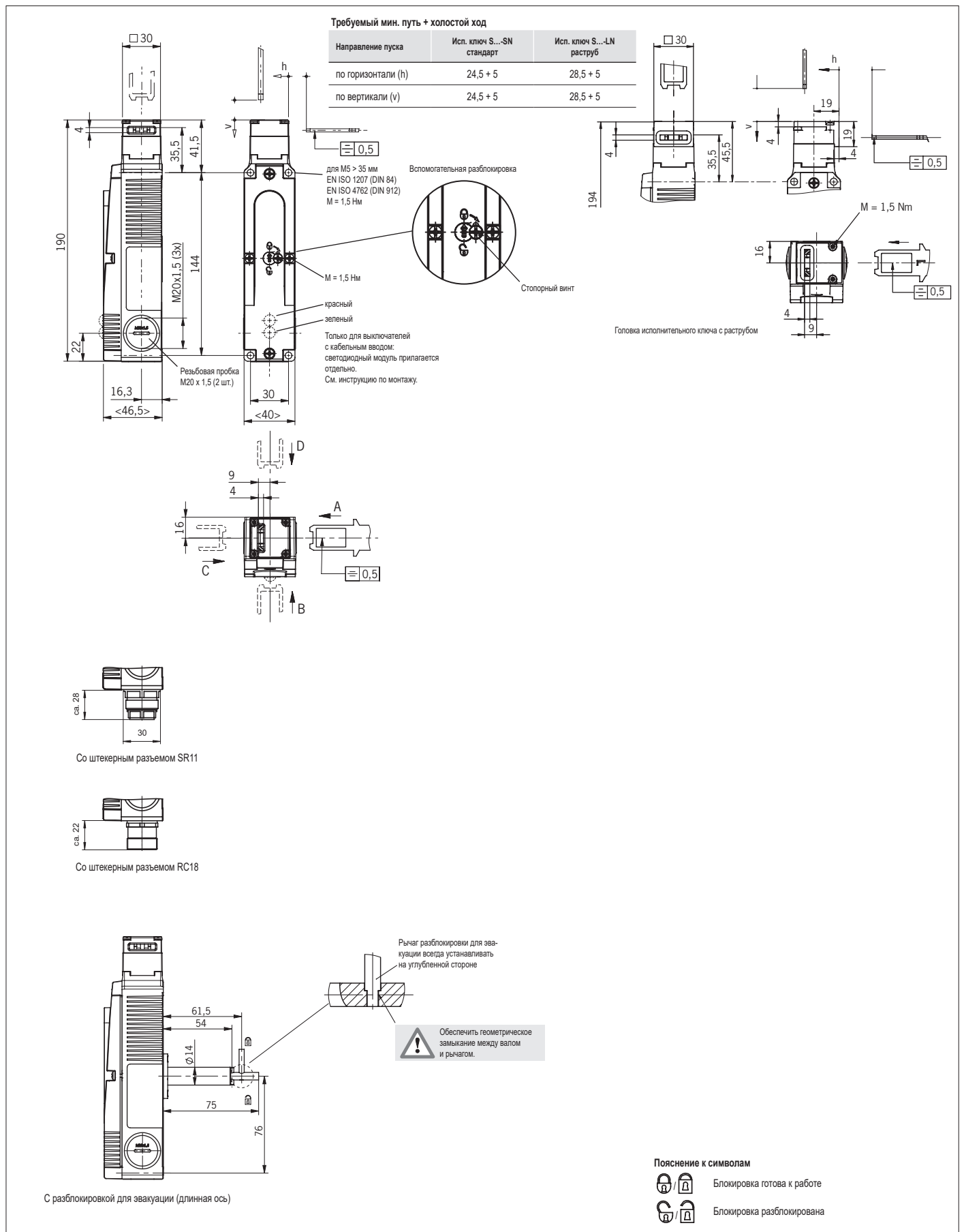
Рис. 2. Размерный чертеж STA... без раструба и STA... с раструбом
