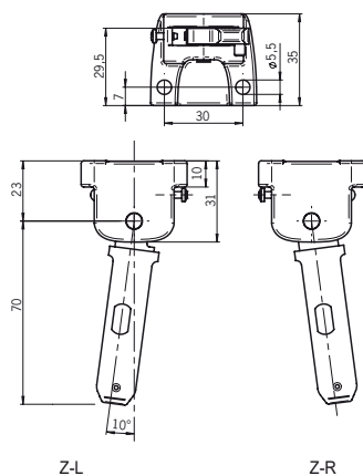
Polimerový ovládač Z-L / Z-R
