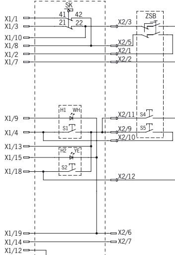
Obrázok 9: TZ..VA-C2199 s osvetlenými tlačidlami a pripojením odsúhlasovacieho spínača
