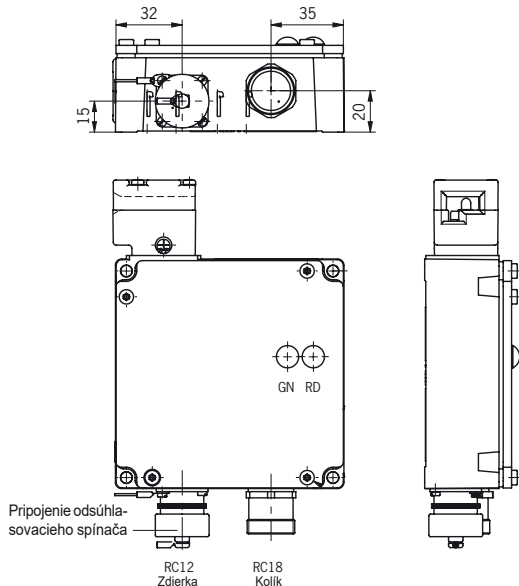
Obrázok 7: TZ..VAB-C1803 s pripojením odsúhlasovacieho spínača
