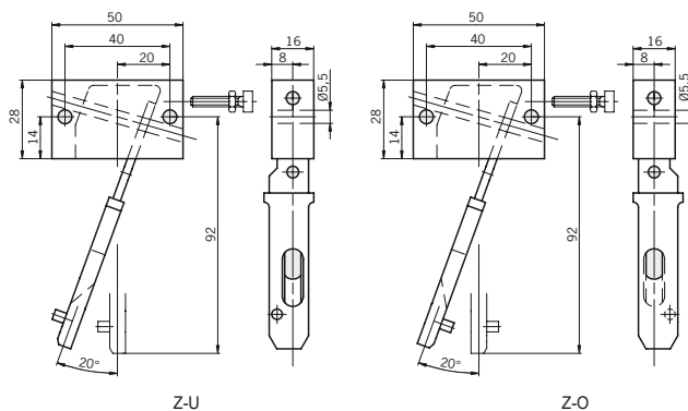
Polimerový ovládač Z-U / Z-O
