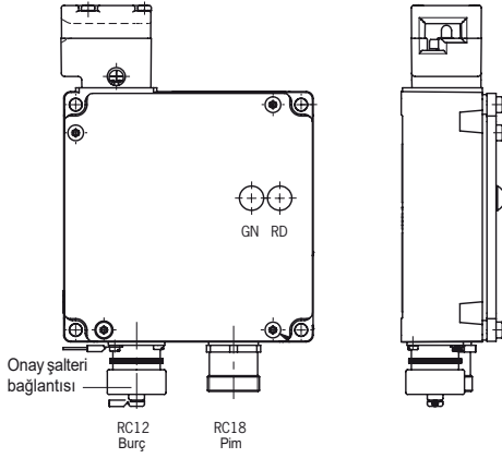
Resim 7: TZ..VAB-C1803, onay şalteri bağlantısı ile
