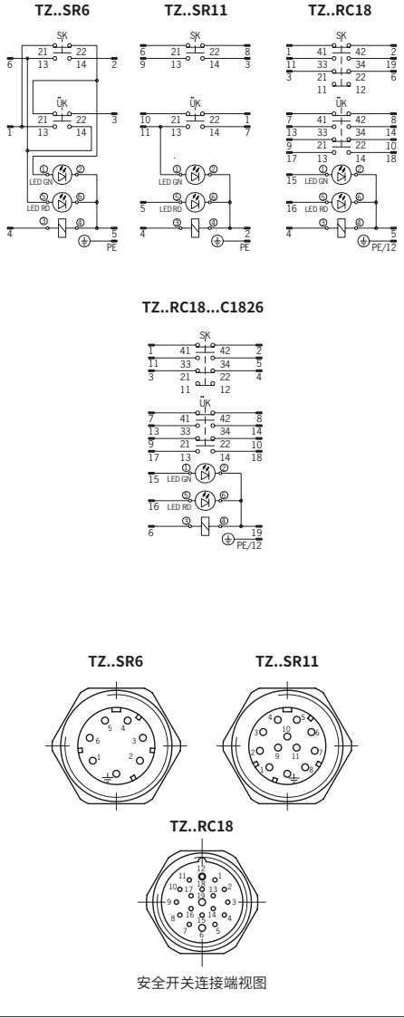
图3：接头分配
