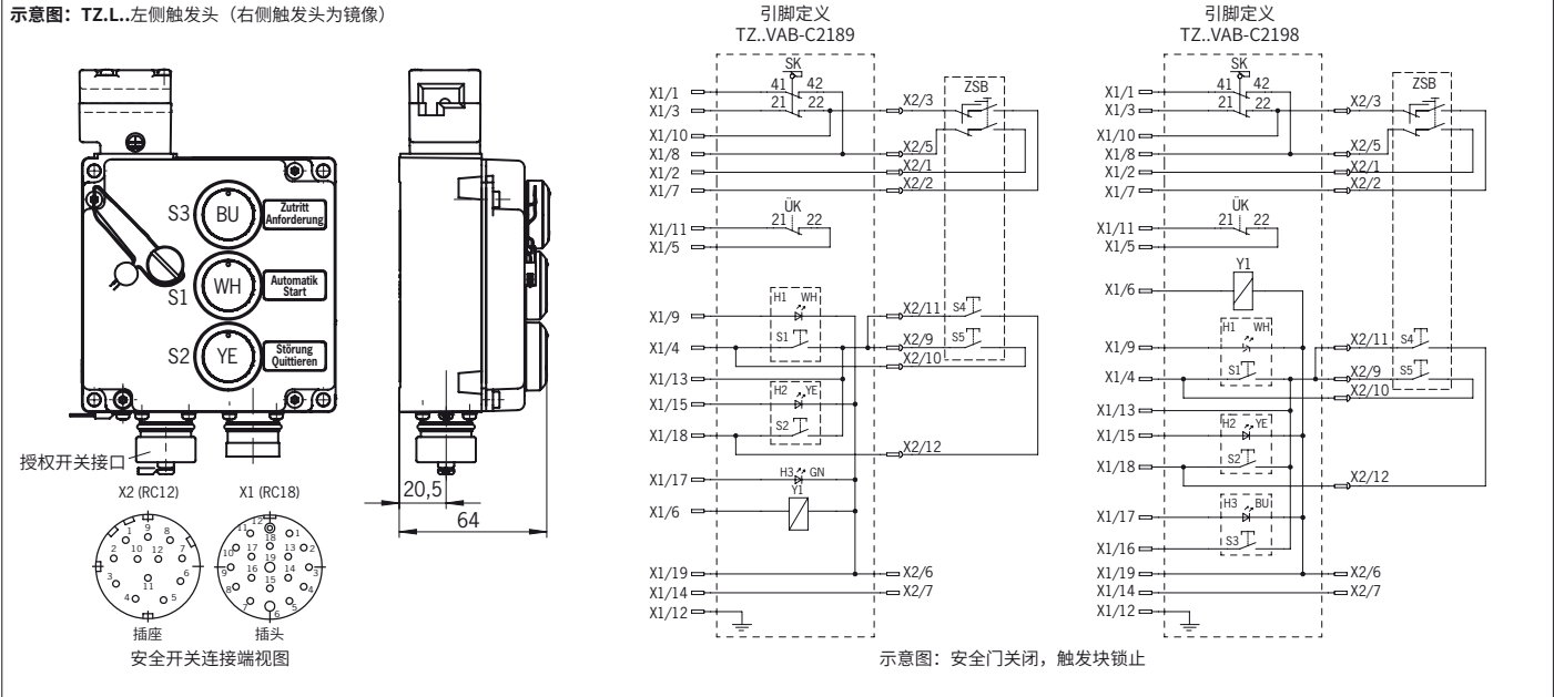
图8: TZ..VAB-C2189/2198, 配有指示灯/发光按钮和授权开关接口
