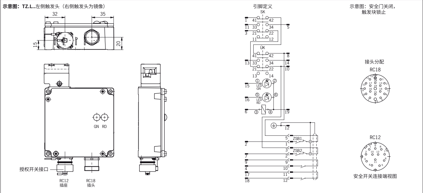
图7: TZ..VAB-C1803, 配有授权开关接口
