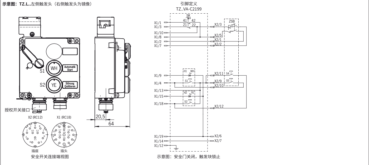
图9: TZ..VA-C2199, 配有发光按钮和授权开关接口
