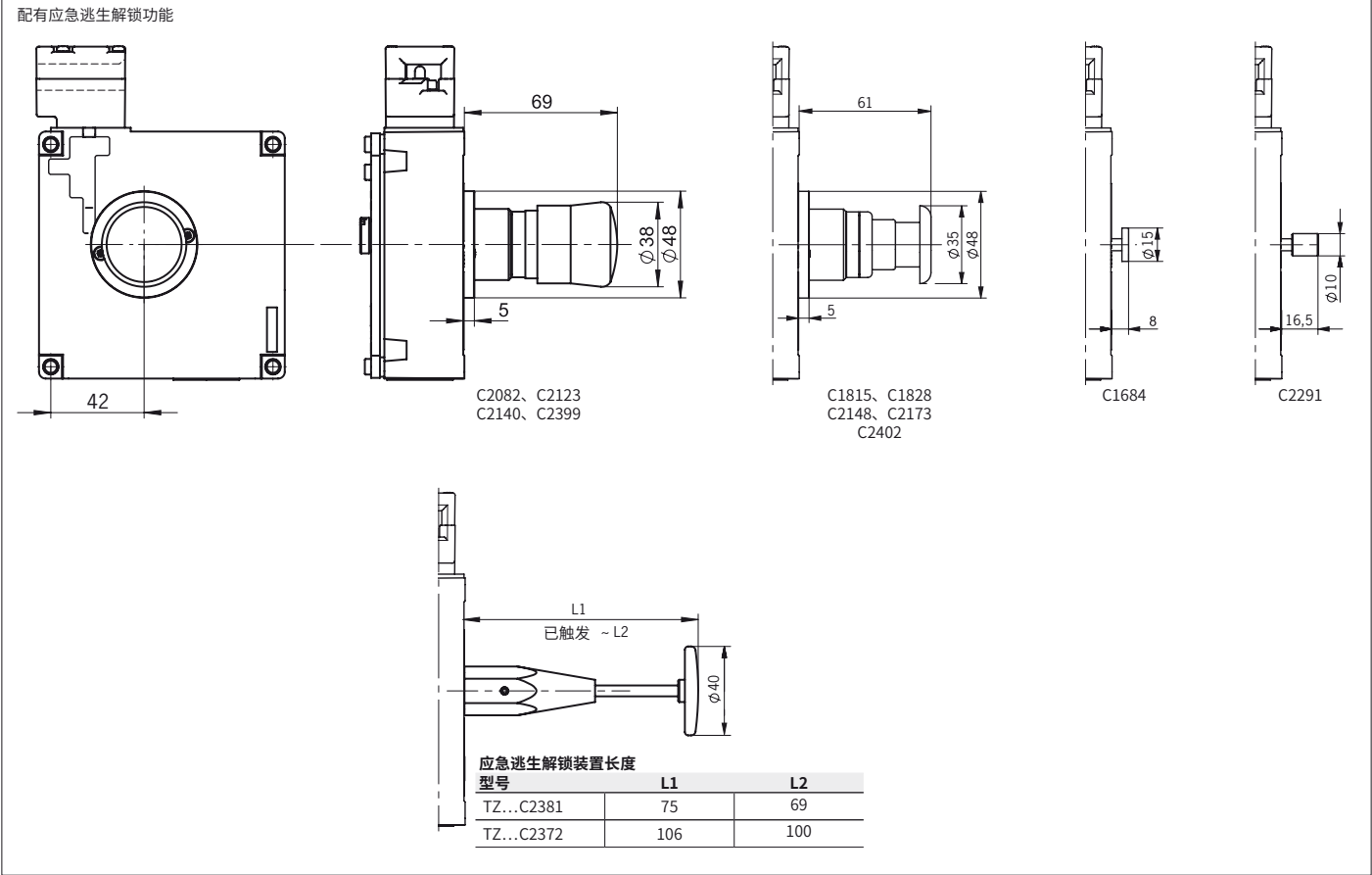
图4: 应急逃生解锁装置的尺寸示意图
