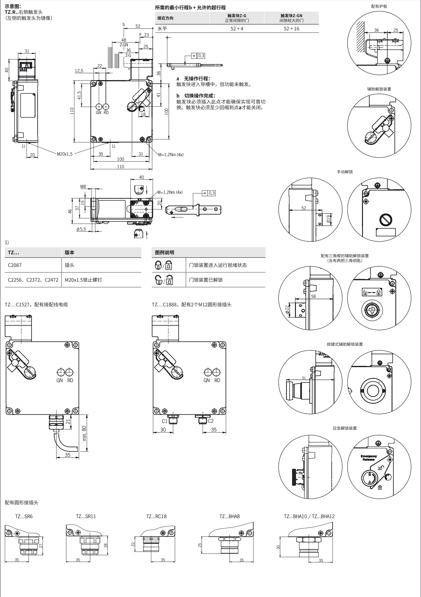
图3: TZ...的尺寸示意图
