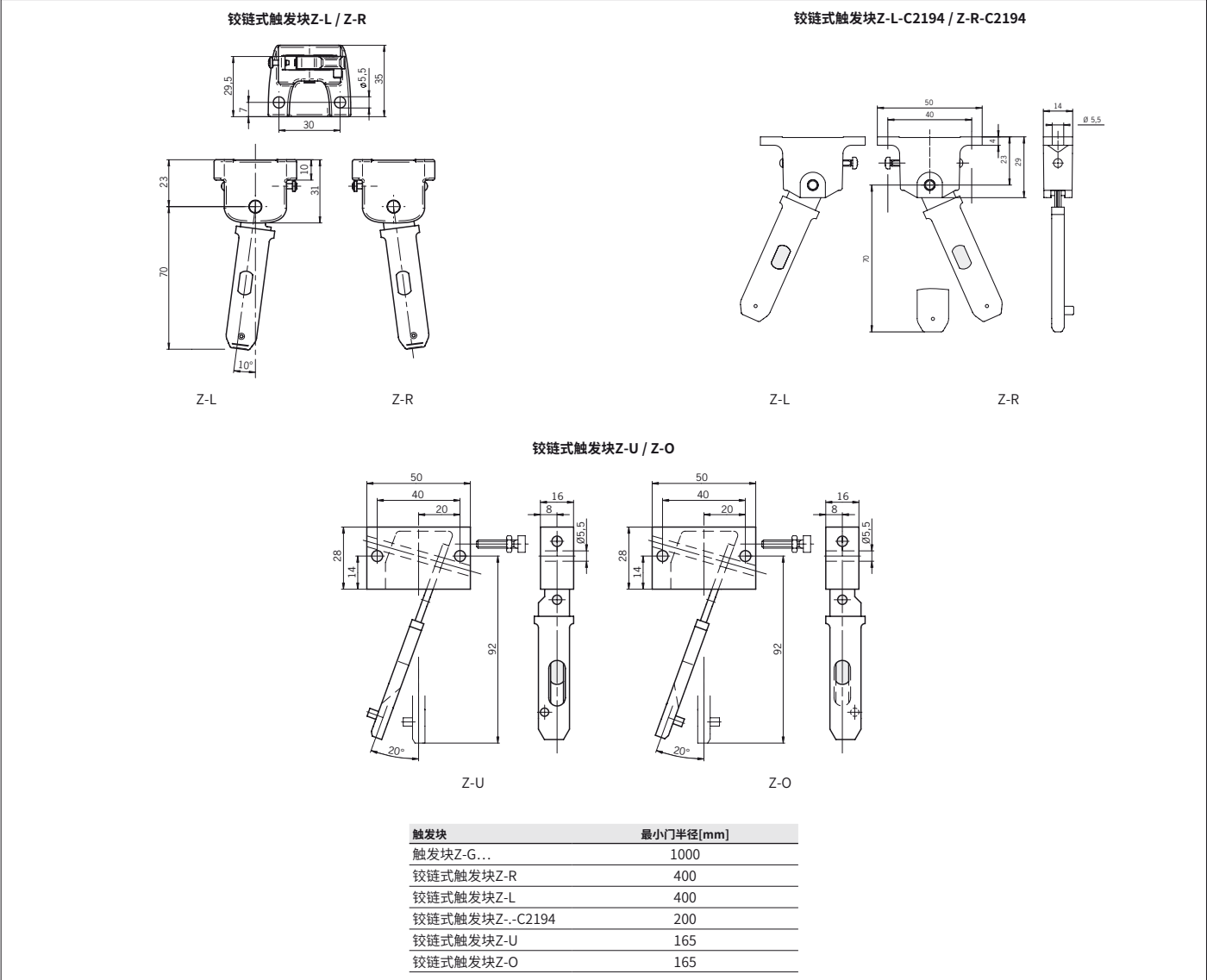
图10：最小门半径
