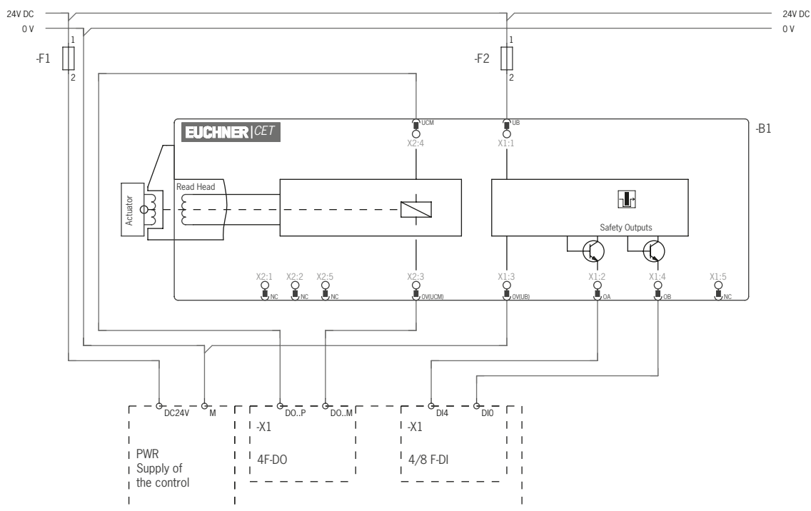
图4: 配线图A, 具有2个M12圆形接头、没有门监控输出的CET 3/4-AP 锁止电磁线圈双通道控制
