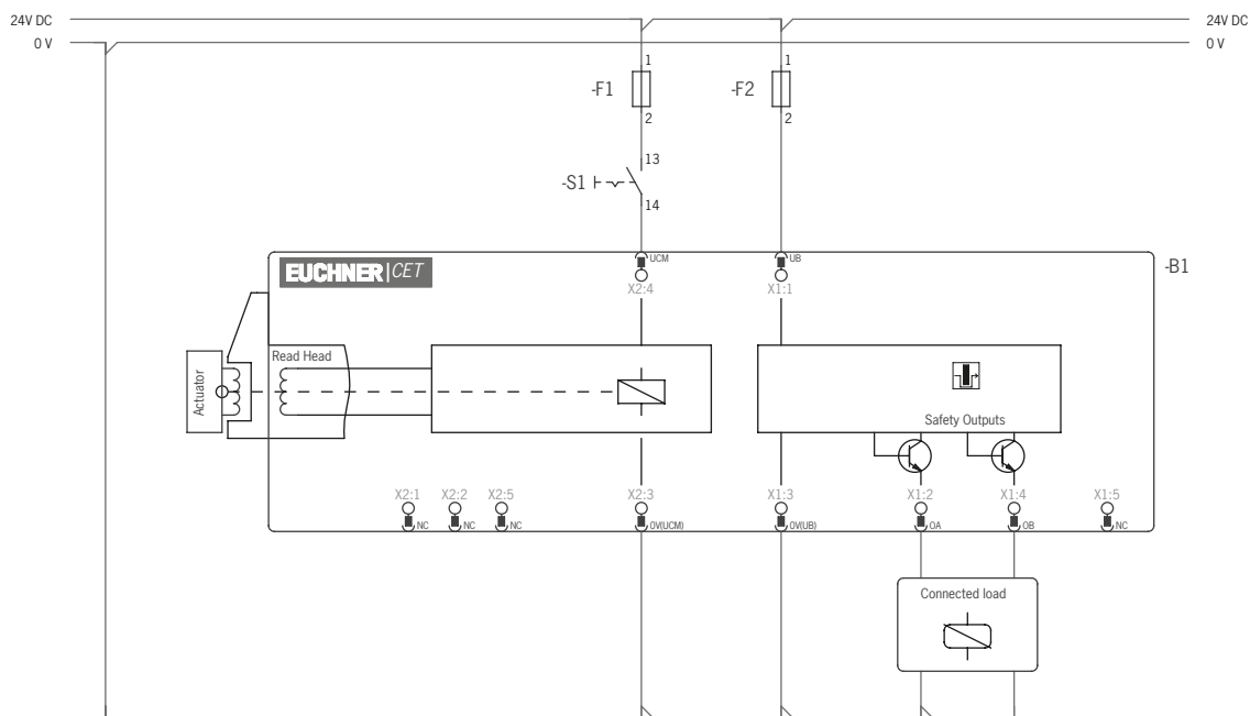
图3: 配线图A, 具有2个M12圆形接头、没有门监控输出的CET 3/4-AP 锁止电磁线圈单通道控制
