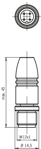
带式插头097645 4针, 插头 (图示相近)
