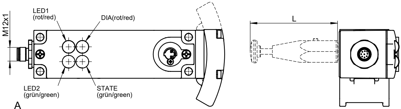
CET...AP... ( 1 x M12 ) Ansicht Steckseite A View plug connection side A
