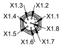
CET...AP... ( 1 x M12 ) Ansicht Steckseite A View plug connection side A
