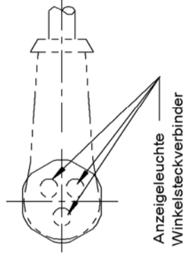
Ansicht "Z"
