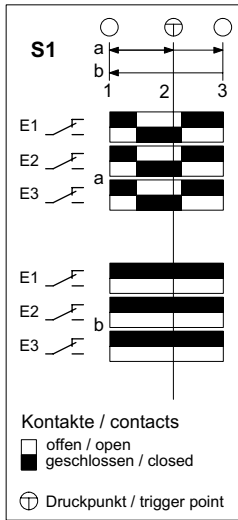
S1: Zustimmtaster enabling pushbutton
