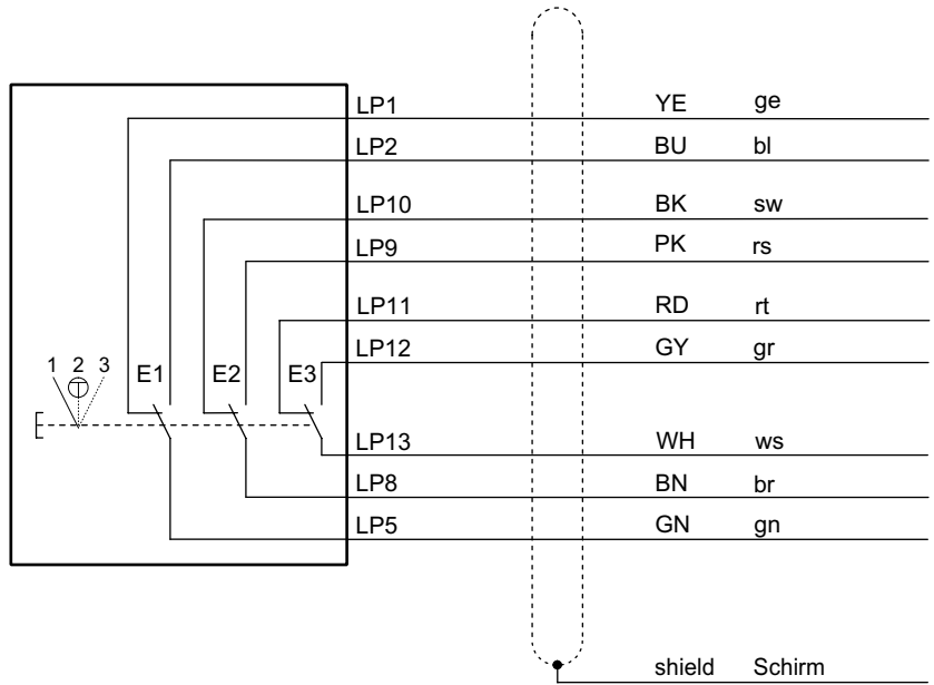
S1: Zustimmtaster enabling pushbutton
