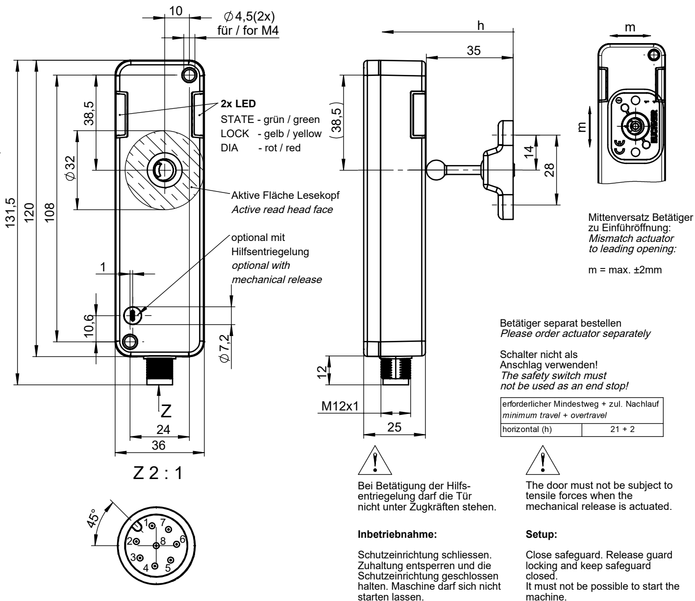
Steckerbelegung Sicherheitsschalter mit Stecker 8-pol. M12x1 (SA) BR Ausgangsfamilie Pin assignment safety switch with connector 8-pole. M12x1 (SA) BR output family
