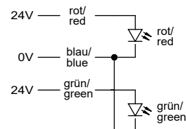
Anschlussplan / Wiring Diagram
