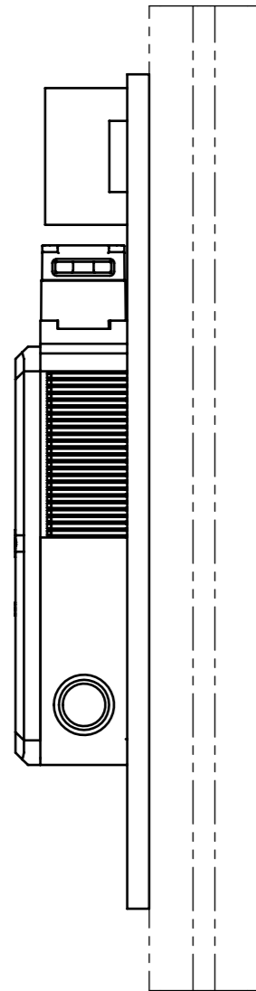
Ansicht B View
