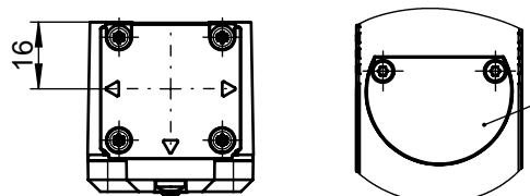
Ansicht / View Y
