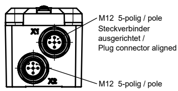
Ansicht / View Z
