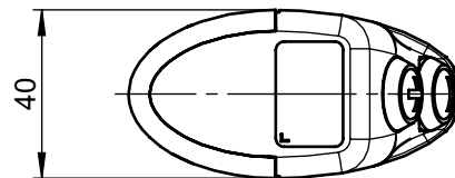
Polbild / Mating face Ansicht Steckseite / View of connection side 1:1
