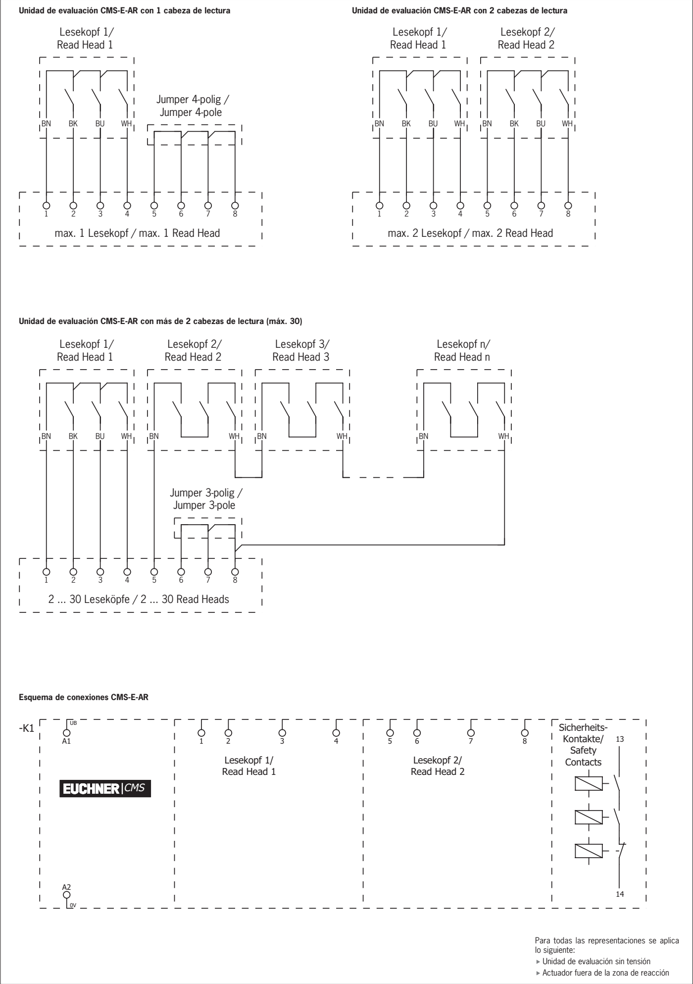
Fig. 2: Esquema de conexiones CMS-E-AR
