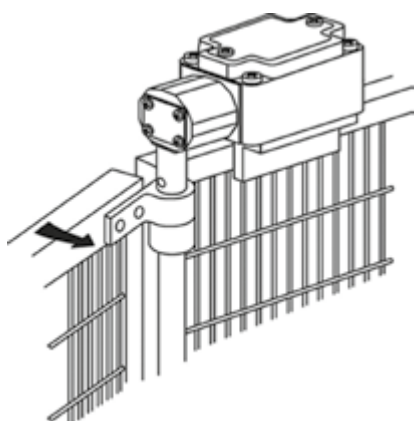
Abb. 35 Bsp. Scharnierschalter
