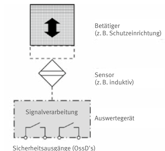
Abb. 14 unkodierter Näherungsschalter
