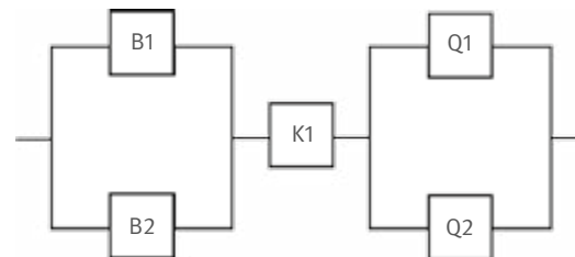
Abb. 53 Stellungsüberwachung beweglicher trennender Schutzeinrichtungen mit Blockschaltbild
