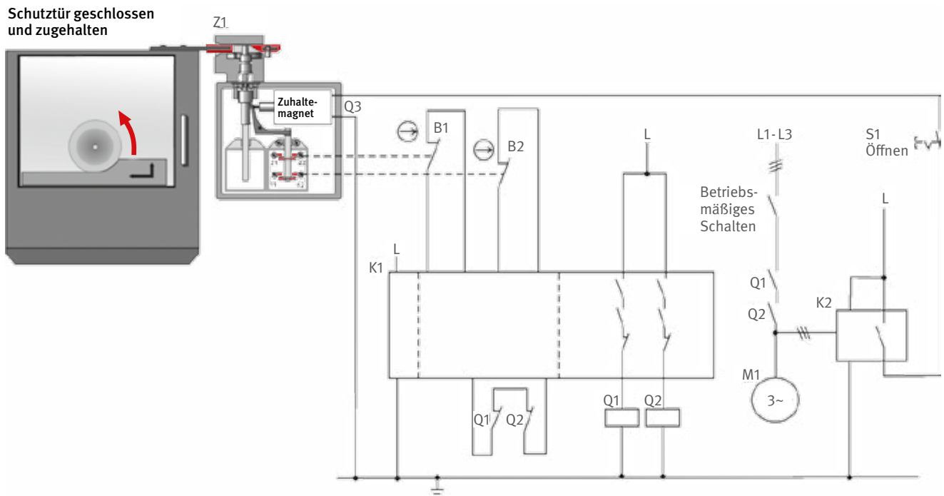
Abb. 54 Stellschaltung für eine bewegliche trennende Schutteinrichtungen
