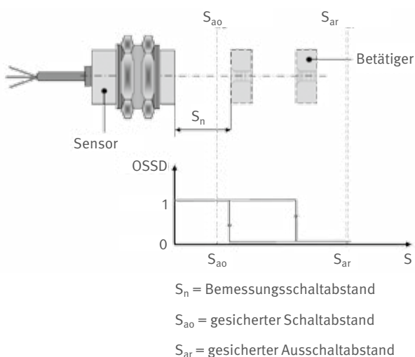
Abb. 18 Schaltabstände
