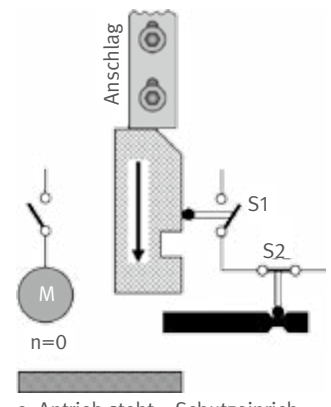
e: Antrieb steht – Schutzeinrichtung nicht geschlossen – Zuhaltung in Sperrstellung aber ohne Sperrfunktion
