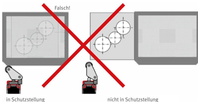
Abb. 31 Unzulässige Anordnung eines Positionsschalters Bauart 1 an einem Schiebeschutzgitter
