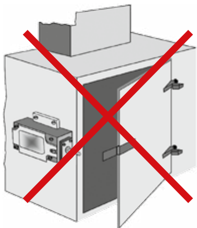
Abb. 33 Unzulässige Anbringung eines Positionsschalters Bauart 1
