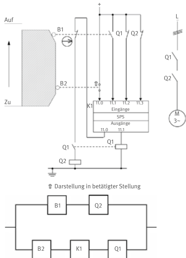
Abb. 52 redundante Stellungsüberwachung einer beweglichen trennenden Schutzeinrichtung in diversitärer Technologie mit Blockschaltbild
