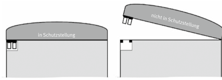
Abb. 36 Stellungenüberwachung einer Schutteinrichtung an der Schließkante
