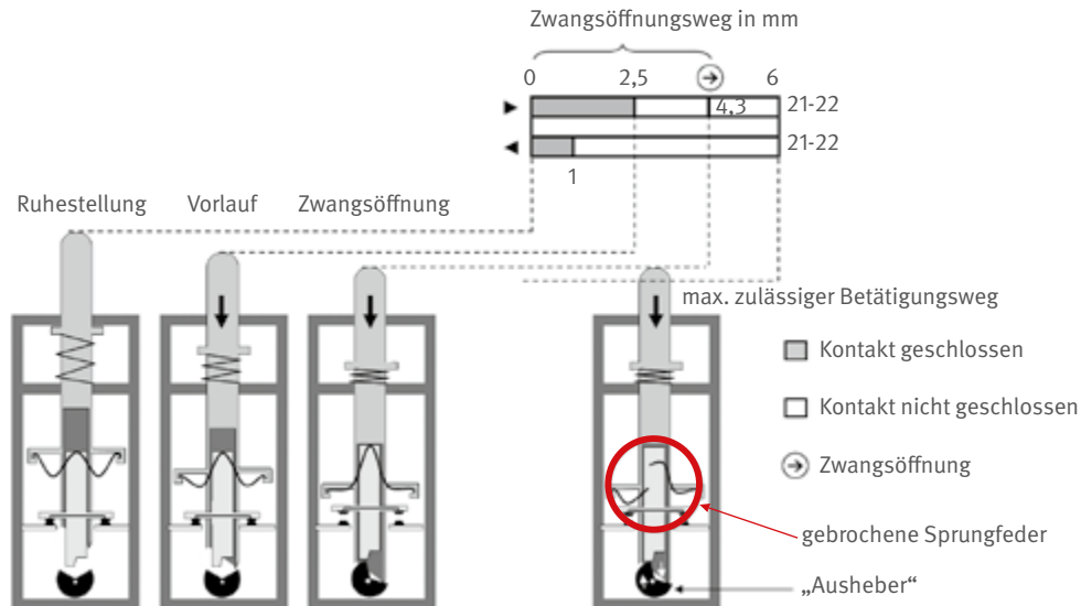
Abb. 13 Zwangsöffnender Schalter mit Sprungfunktion (nur Öffnerkontakt dargestellt) mit Schaltwegdiagramm
