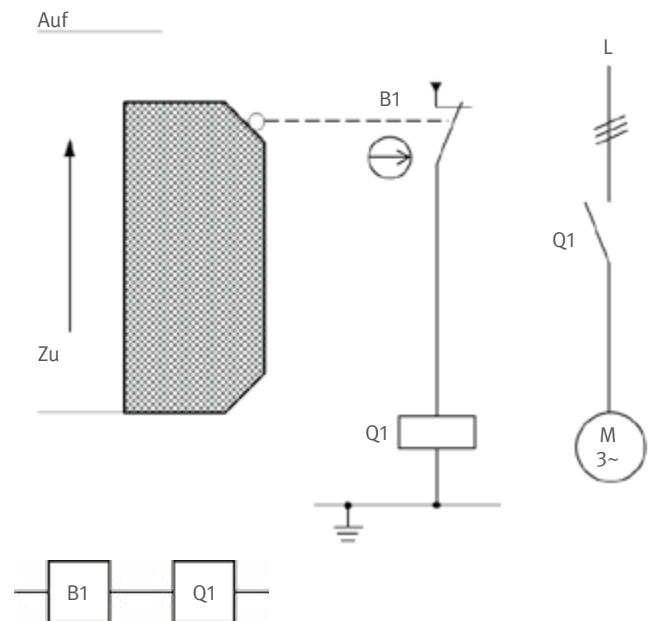
Abb. 51 Stellungsüberwachung einer beweglichen trennenden Schutzeinrichtung mit Blockschaltbild
