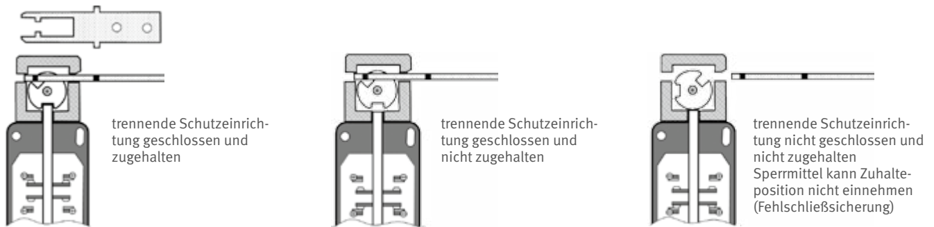
Abb. 20 Zuhaltung mit Fehlschließesicherung
