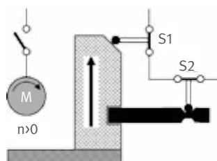
b: Antrieb abgeschaltet (Nachlauf) – Schutzeinrichtung geschlossen – Zuhaltung gesperrt
