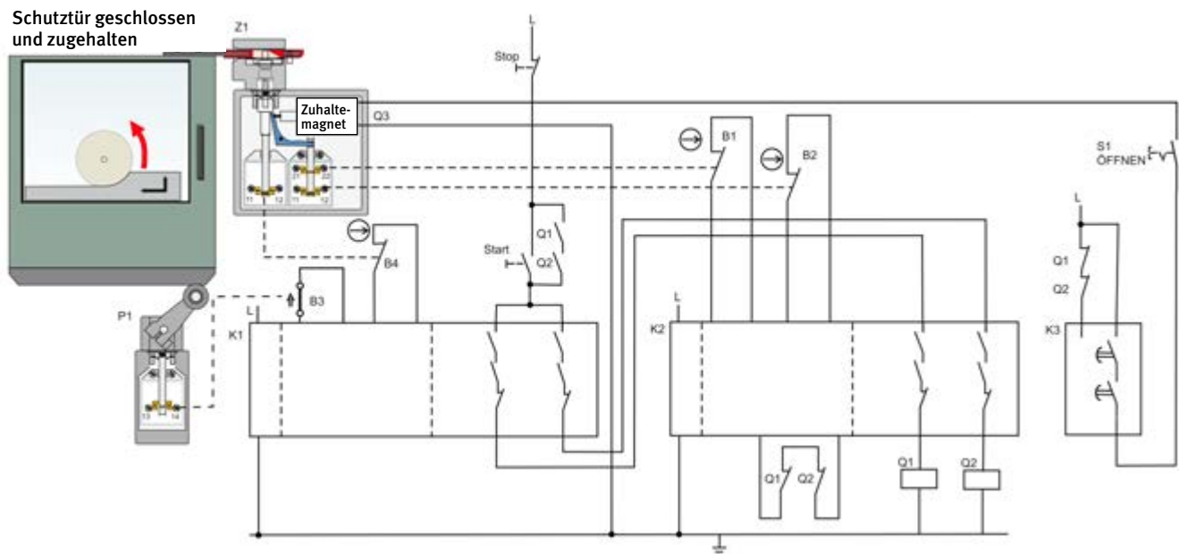
Abb. 57 Stellschaltung einer beweglichen trennenden Schutteinrichtung mit Zuhaltung
