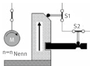
a: Antrieb eingeschaltet – Schutzeinrichtung geschlossen – Zuhaltung gesperrt
