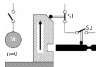
c: Antrieb steht – Schutzeinrichtung geschlossen – Zuhaltung sperrt nicht
